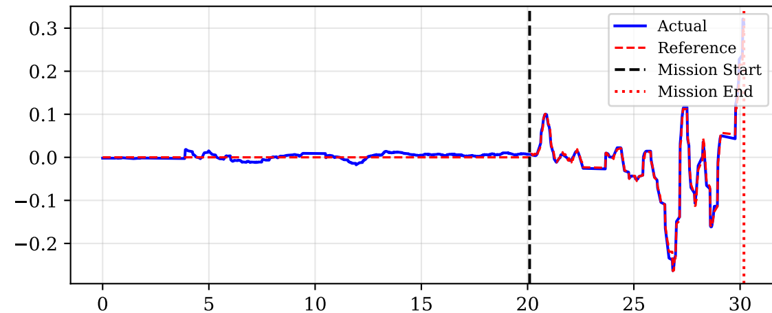
Roll [rad]
