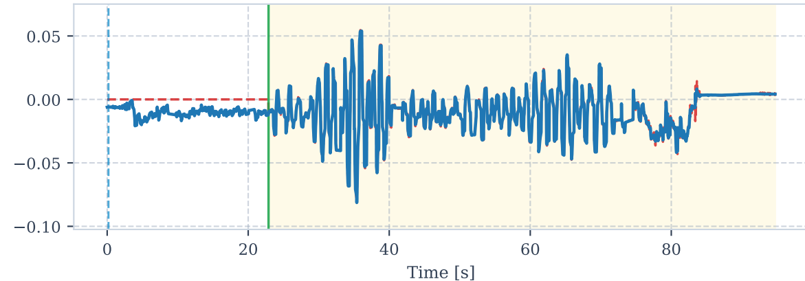
Roll [rad]
