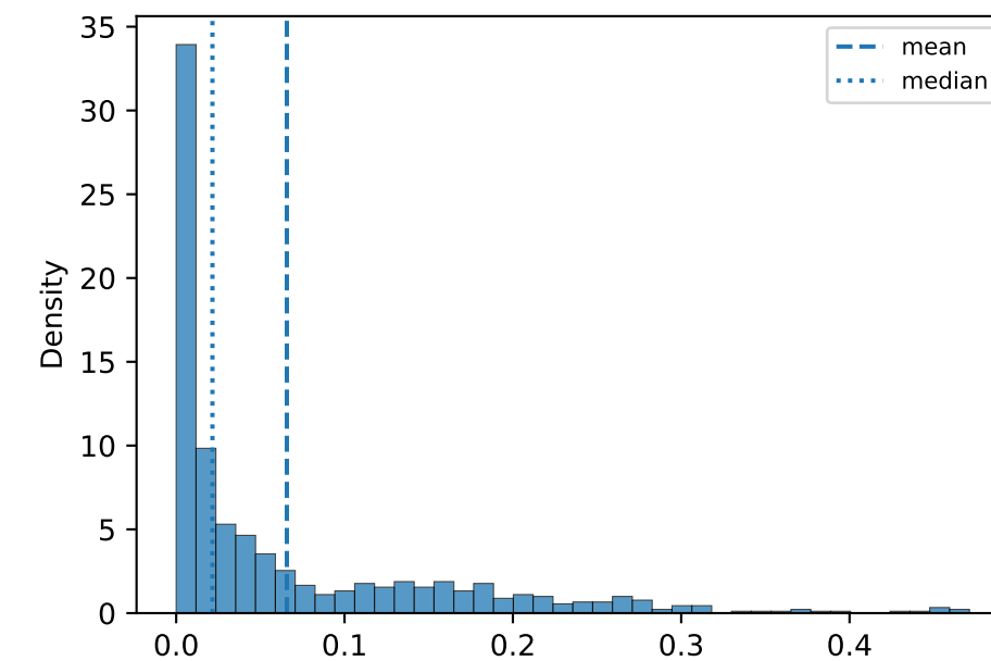
API
