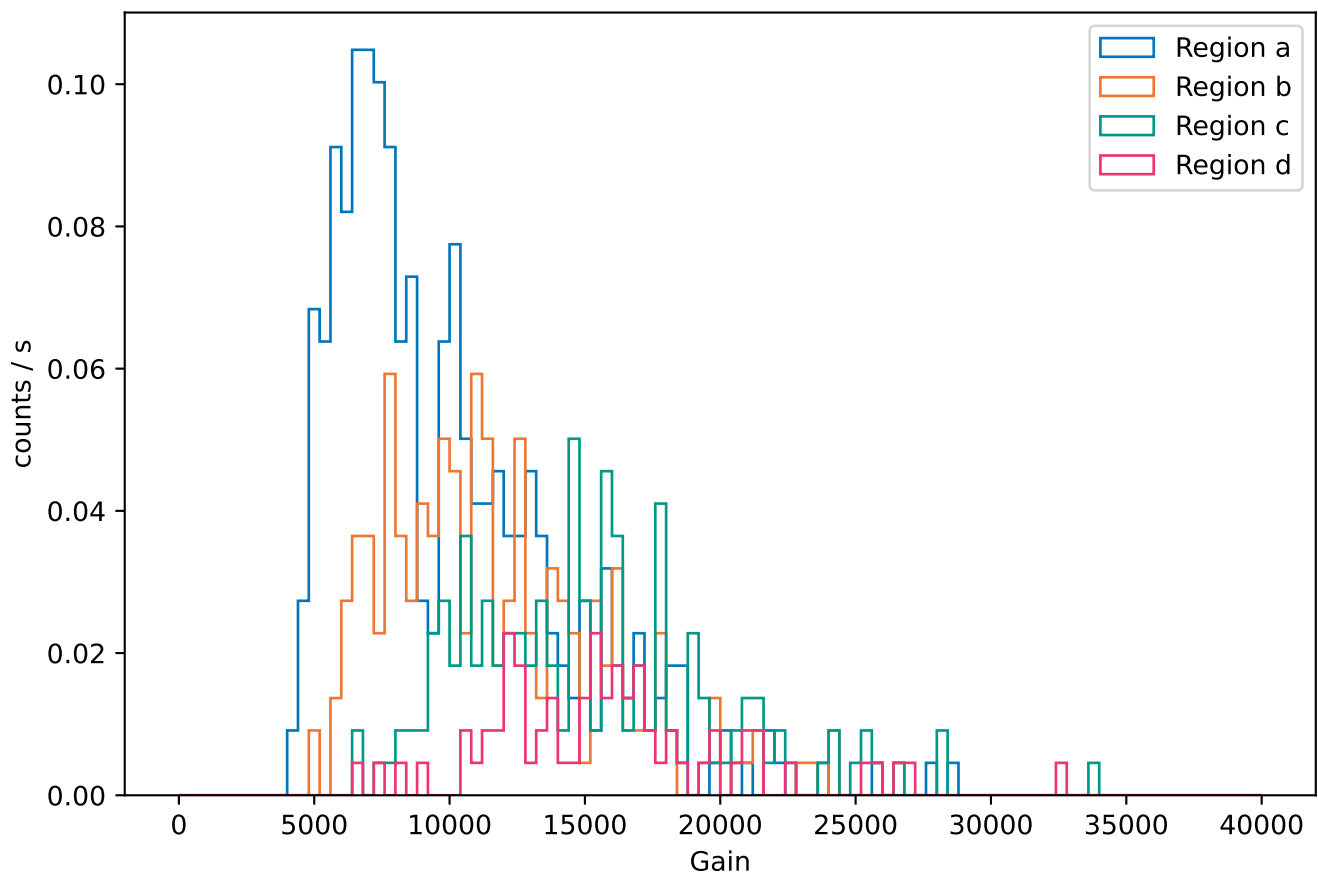
Dataset: 760V
