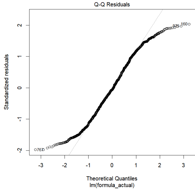
Figura 2. Gráfico Cuantil-Cuantil (Q-Q Plot) de los residuales del modelo.
