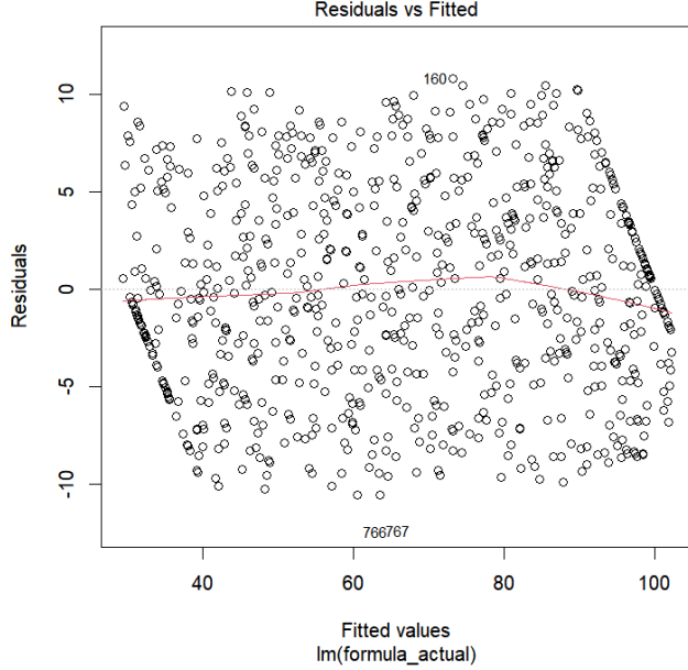
Figura 3. Gráfico de residuales frente a valores ajustados para la verificación de varianza constante.
