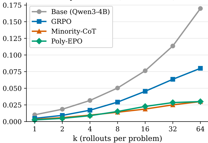
BeyondAIME (n=100, OOD)
