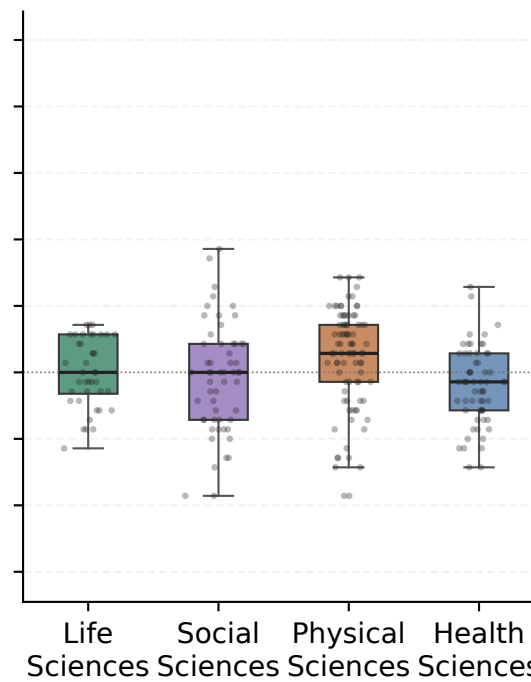
PCA D80
