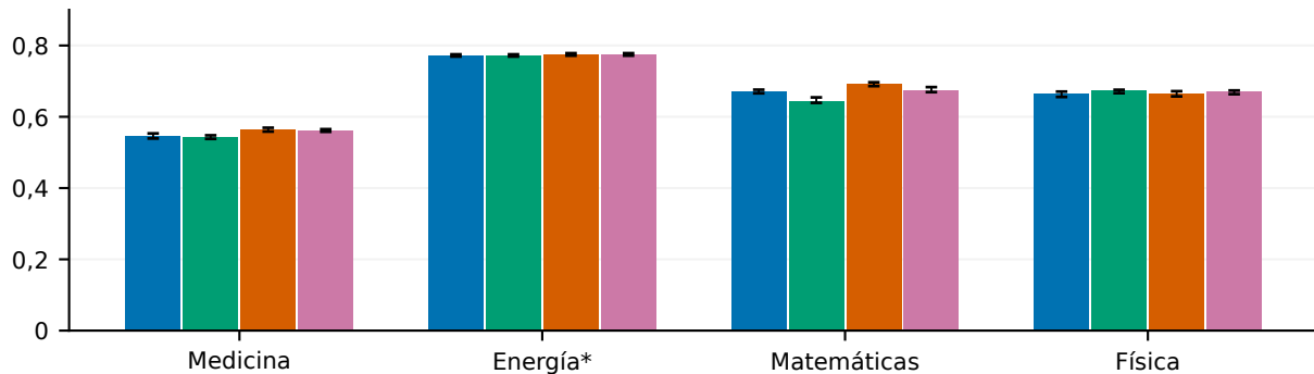
A Forma: CKA corregida
