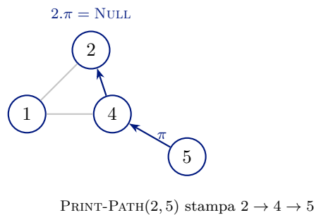
Figura 30. Catena dei predecessori da BFS per ricostruire il cammino minimo 2 \rightarrow 4 \rightarrow 5 .
