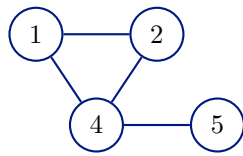
Figura 22. Grafo non orientato d'esempio e liste di adiacenza.
