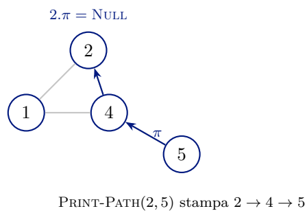
Figura 30. Catena dei predecessori da BFS per ricostruire il cammino minimo 2 \rightarrow 4 \rightarrow 5 .
