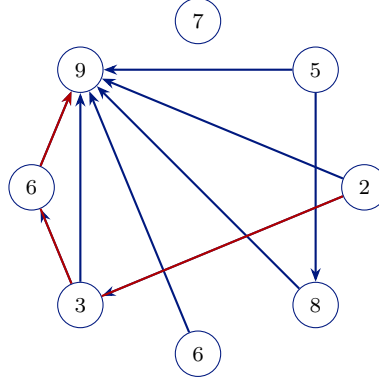
Figura 19. DAG per a = \langle 5, 2, 8, 6, 3, 6, 9, 7 \rangle : cammino massimo 2 \rightarrow 3 \rightarrow 6 \rightarrow 9 (lunghezza 4).
