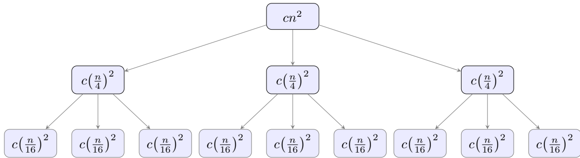
Figura 9. Albero di ricorsione per T(n) = 3T(\lfloor n/4 \rfloor) + \Theta(n^2) .
