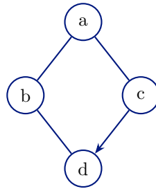
Figura 26. DAG per l'ordinamento topologico (architettura delle slide).
