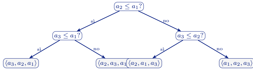
Figura 13. Albero di decisione di INSERTIONSORT su n = 3 (schema parziale delle foglie).
