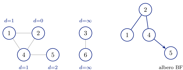
Figura 24. Grafo con distanze finali da s=2 (sinistra) e albero BF con archi \pi (destra).
