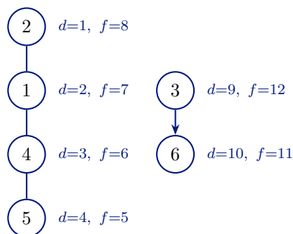
Figura 25. Foresta DF dell'esempio e tempi d/f (schema delle slide).
