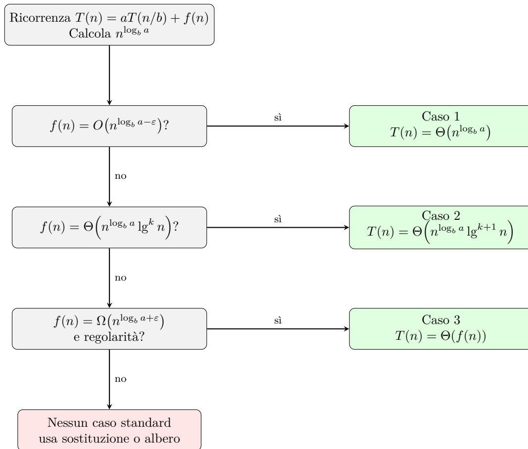
Figura 10. Diagramma di flusso per l'applicazione del Teorema dell'Esperto.
