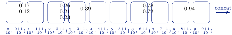
Figura 16. Schema esecutivo di BUCKETSORT ( n = 10 ): inserimento negli intervalli e concatenazione.
