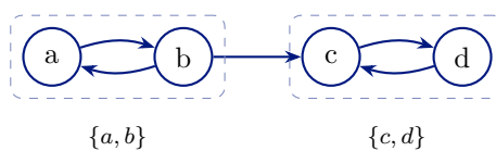
Figura 28. Grafo orientato G e componenti fortemente connesse (esempio SCC delle slide).
