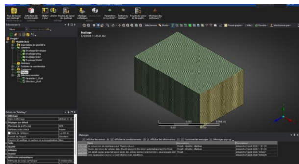
Maillage volumique du domaine — Ansys Meshing
