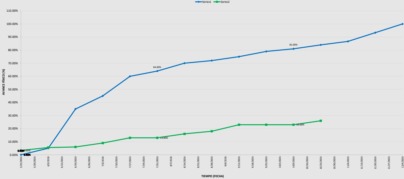
CURVA S DE AVANCE FISICO
