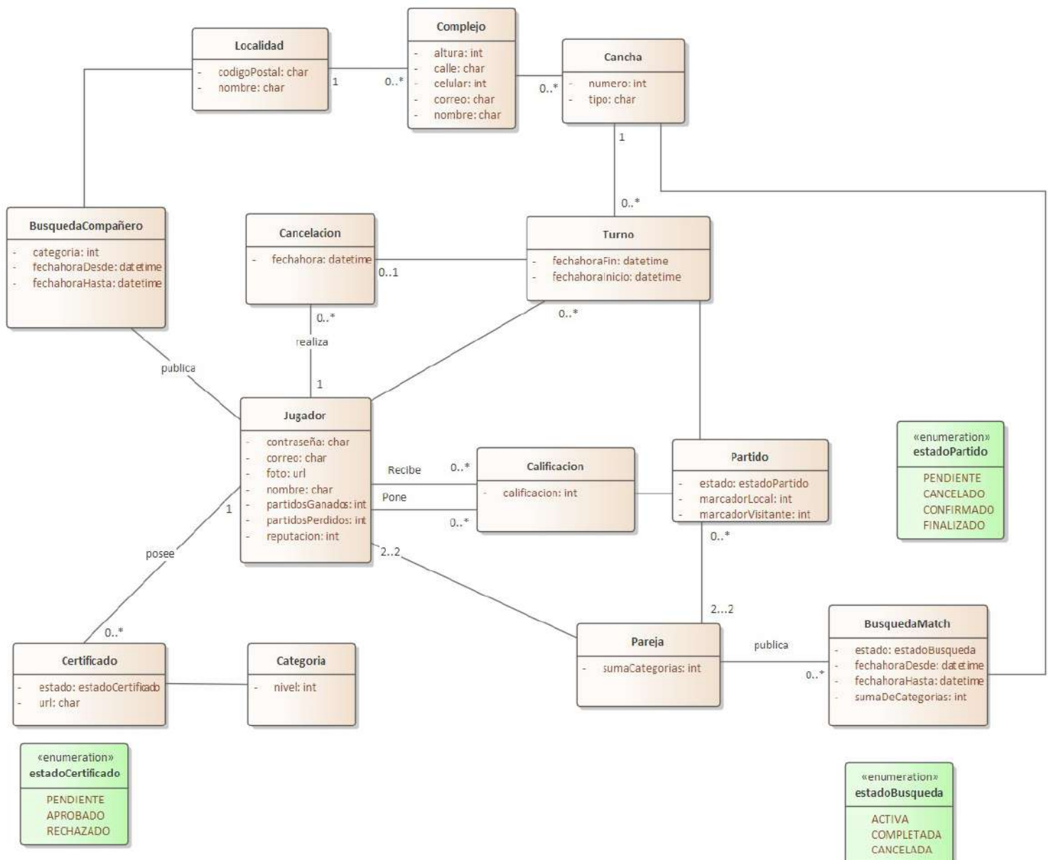
class DiagramaDeClasesDeDominio
