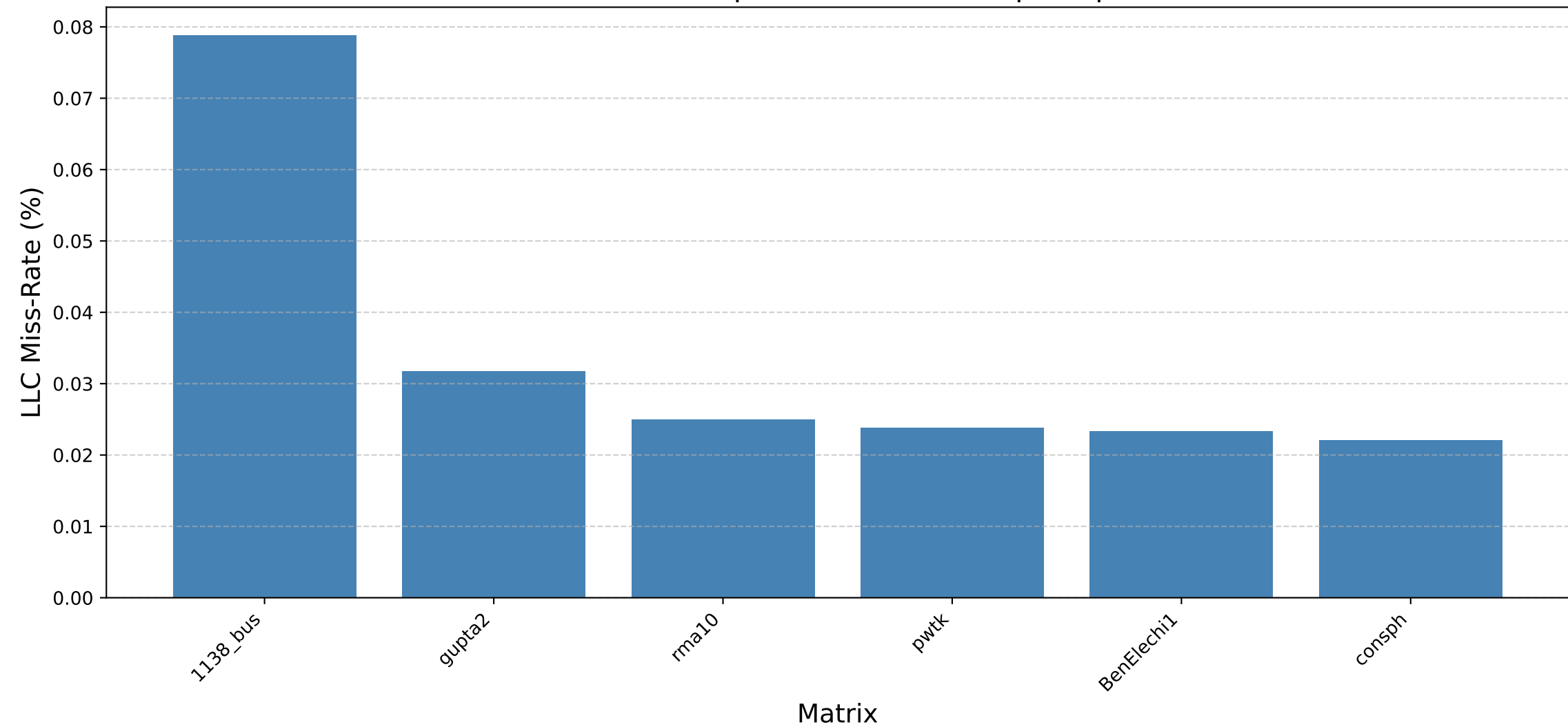
LLC Miss-Rate (%) per Matrice — dati perf (parallel)
