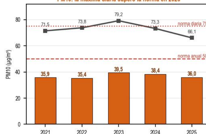
\text{PM}_{10} : la máxima diaria superó la norma en 2023
