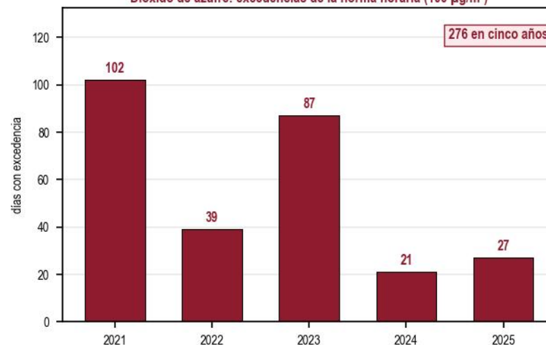
Dióxido de azufre: excedencias de la norma horaria ( 100 \mu\text{g}/\text{m}^3 )
