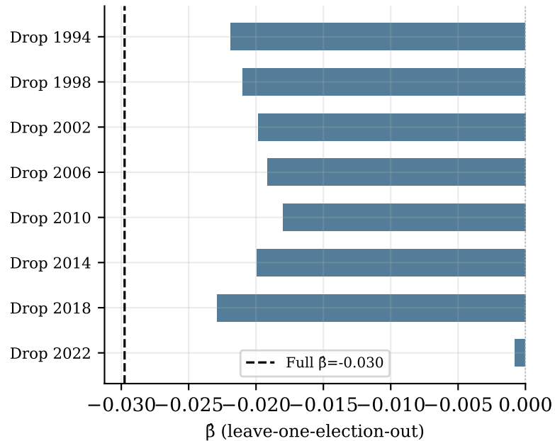
Midterms (PADD): LOEO
