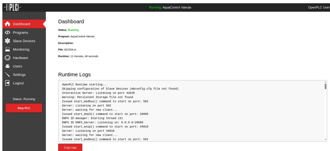
Figura 2. Panel de OpenPLC con el programa AquaControl Valvula en ejecución.
