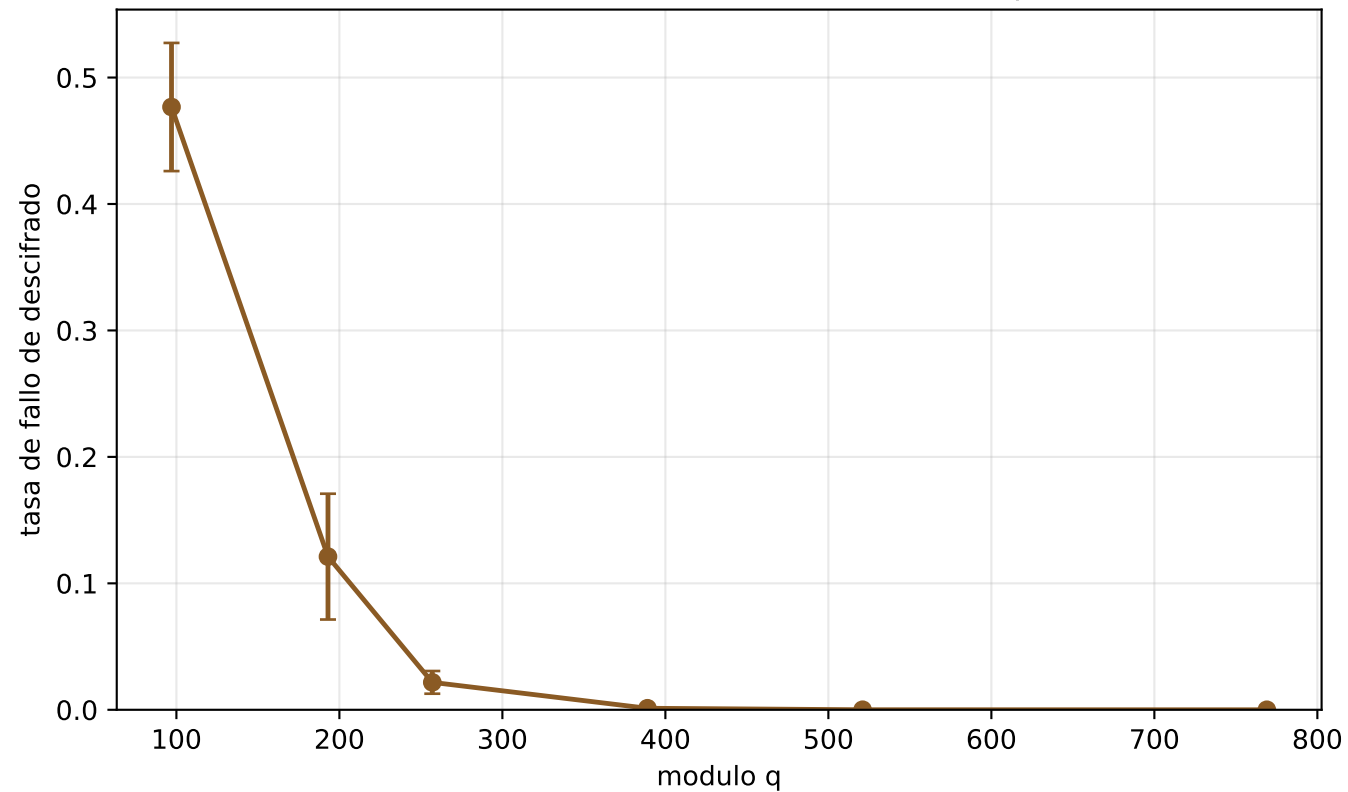
Fallo de descifrado frente al modulo q
