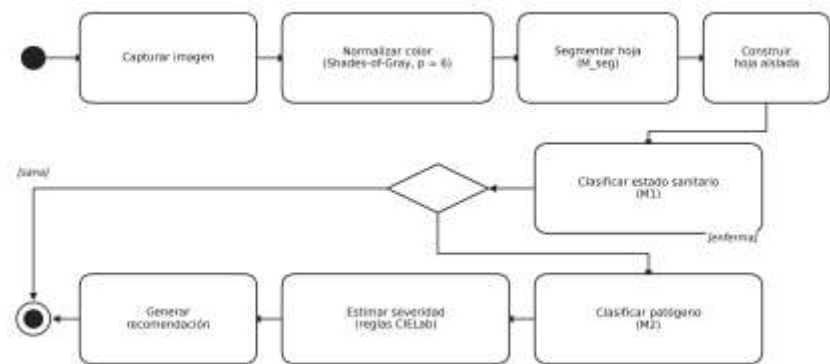
Figura 1. Diagrama de Actividad del Sistema: Normalización Cromática, Segmentación Hoja–Fondo, Clasificación en Cascada y Estimación de Severidad por CIELab.
