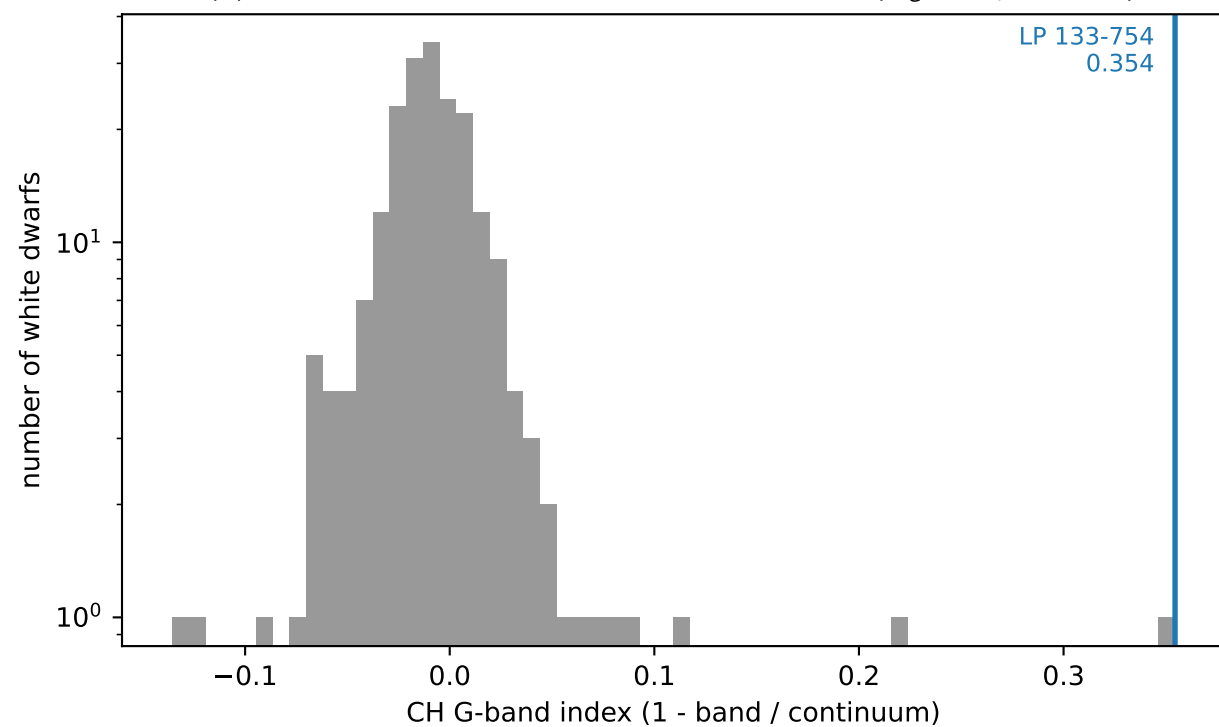
(d) CH index of 208 cool SDSS-V DA white dwarfs ( M_G > 14 , S/N \geq 6 )
