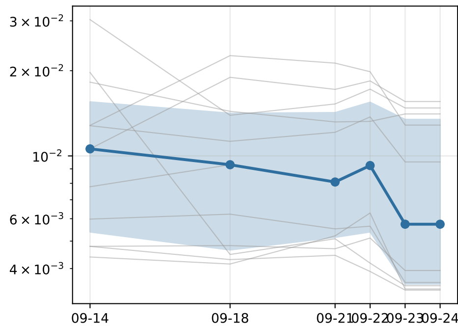
ancilla MCM readout error
