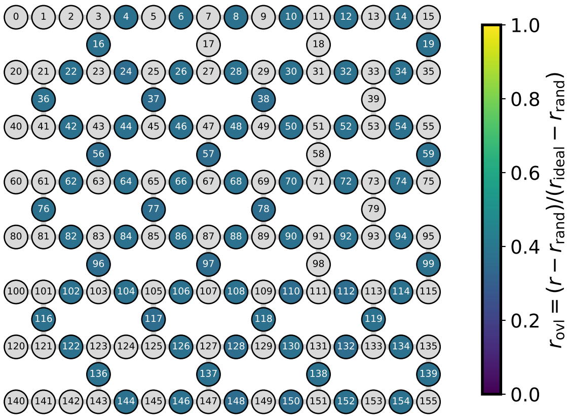
ibm_boston - quality per ancilla, n_data = 60, p = 6
