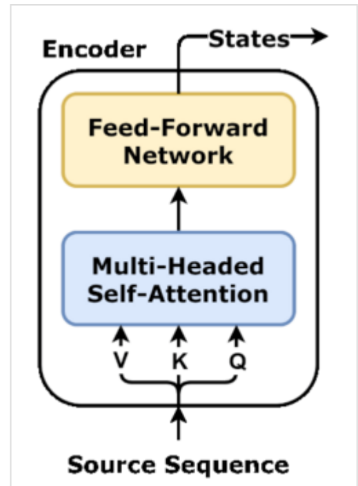
One encoder layer
