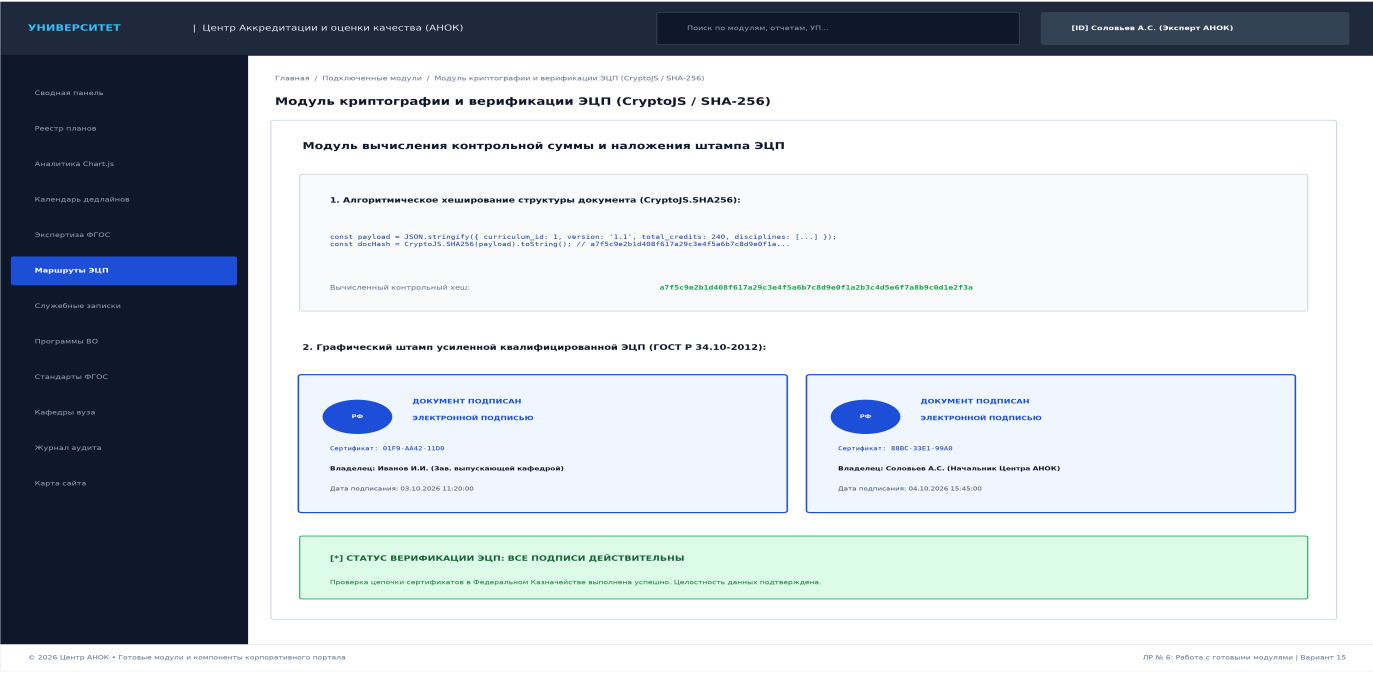
Рисунок 4 — Модуль криптографического хеширования SHA-256 и штампа ЭЦП по ГОСТ
