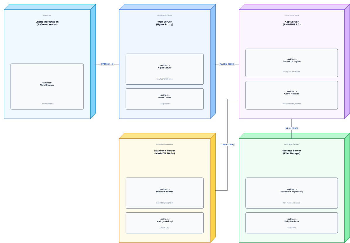
Рис. 4. UML диаграмма развертывания веб-портала
