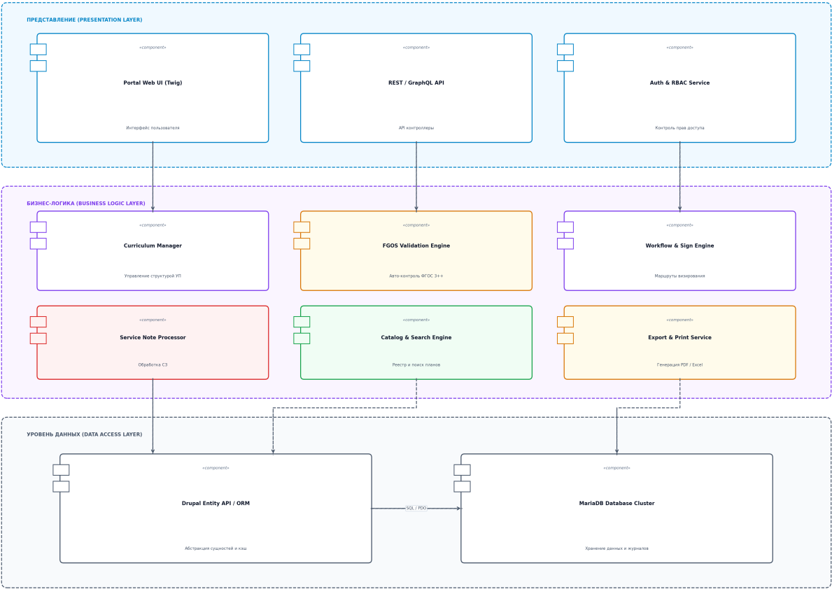
Рис. 3. UML диаграмма компонентов веб-портала
