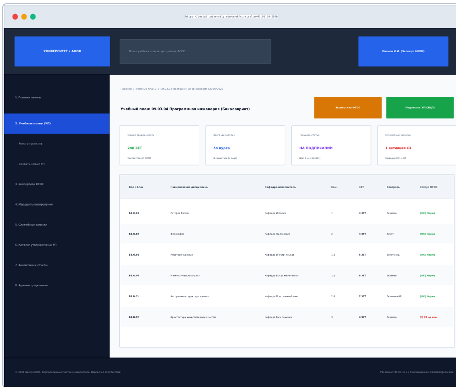
Рисунок 1 — Каркас и структура шаблона дизайна портала (Wireframe Layout)
