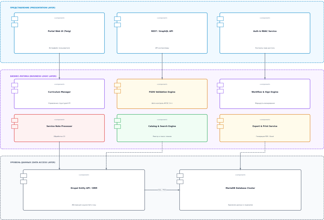
Рисунок 1 — Диаграмма компонентов
