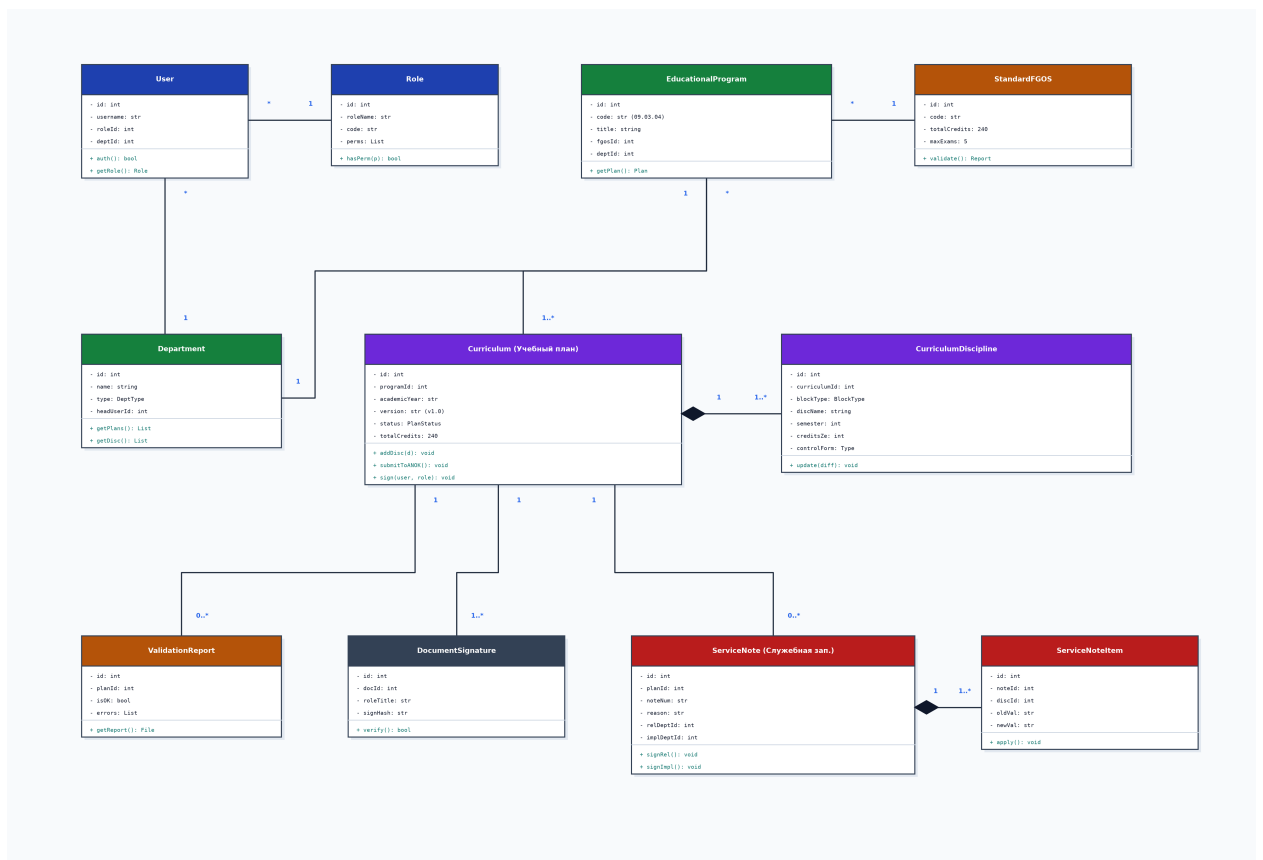
Рисунок 3 — Диаграмма классов
