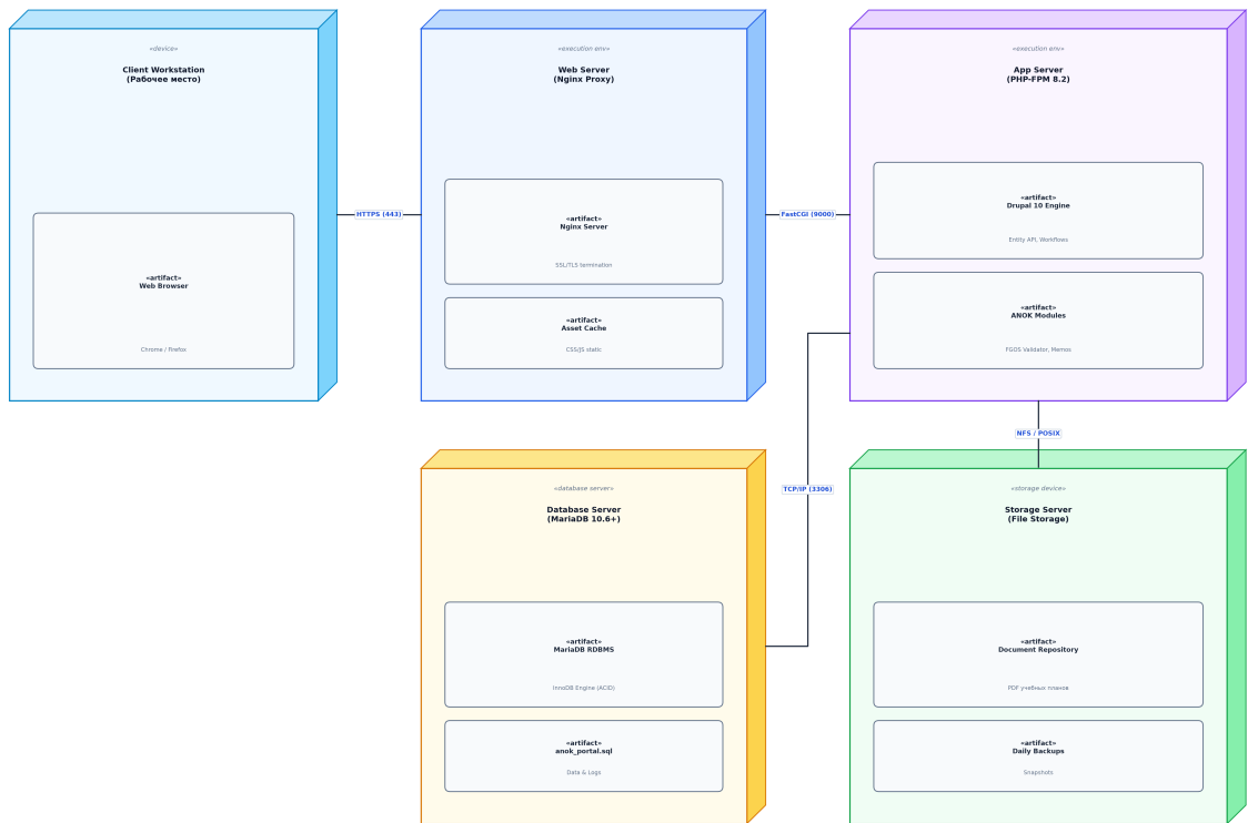
Рисунок 2 — Диаграмма развёртывания
