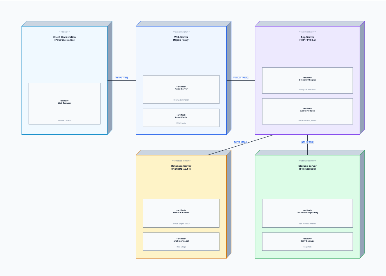
Рис. 4. UML диаграмма развертывания веб-портала
