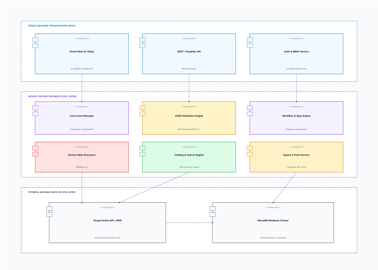
Рис. 3. UML диаграмма компонентов веб-портала
