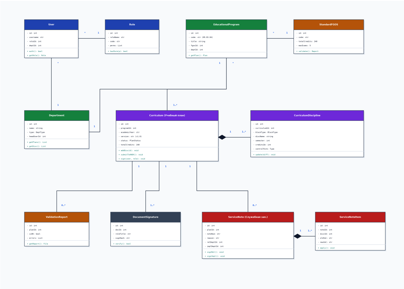
Рис. 1. UML диаграмма классов корпоративного портала (Модуль АНОК)
