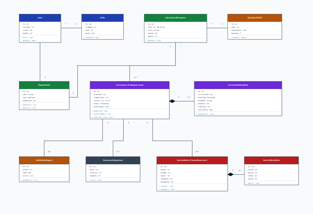
Рисунок 4 — Диаграмма классов
