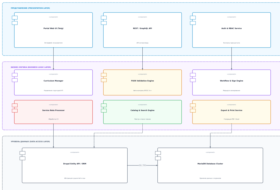
Рисунок 1 — Архитектура проекта
