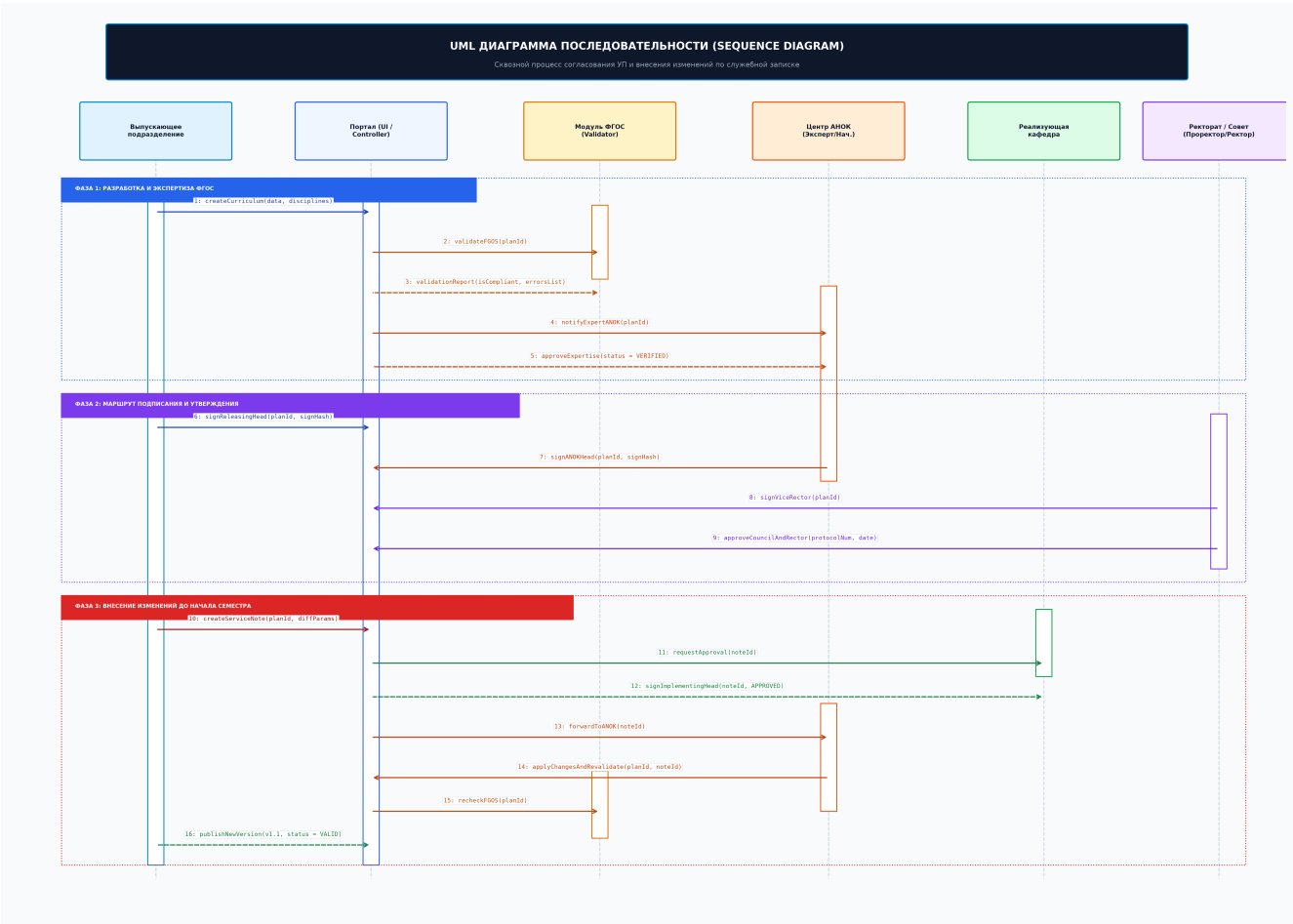
Рис. 2. UML диаграмма последовательности сквозного процесса
