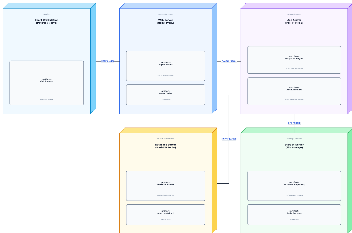
Рисунок 2 — Диаграмма развёртывания
