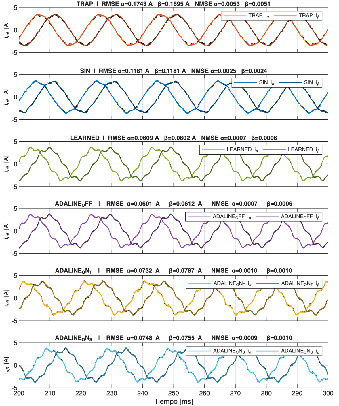
Figura 5.5: Seguimiento de corriente en \alpha\beta durante los últimos 100 ms del escenario con observador (referencia en línea discontinua). Las referencias de los métodos con forma de onda aprendida son no senoidales: contienen los armónicos que (3.6) exige para sostener un par constante con la BEMF real del motor.
