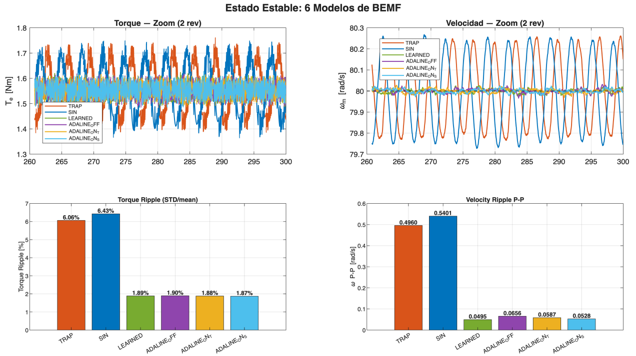
Figura 5.2: Régimen permanente con supervisión ideal. Arriba: par y velocidad sobre dos revoluciones eléctricas; TRAP y SIN exhiben la pulsación periódica que los métodos con forma de onda aprendida no tienen. Abajo: rizo de par y rizo de velocidad pico a pico por método.
