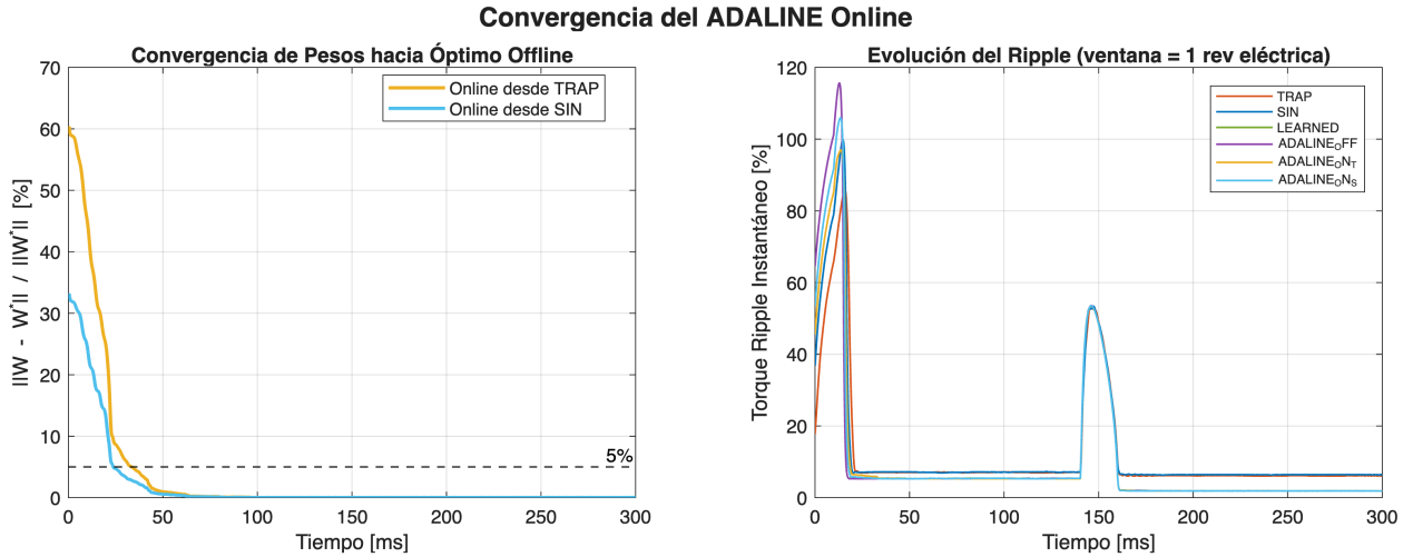
Figura 5.3: Convergencia del ADALINE en línea con supervisión ideal. Izquierda: error relativo de pesos \|\mathbf{W} - \mathbf{W}^*\|_F / \|\mathbf{W}^*\|_F para las dos inicializaciones; ambas cruzan el 5 % en 25–35 ms. Derecha: rizo de par instantáneo (ventana móvil de una revolución eléctrica); tras la convergencia, los métodos en línea se asientan en el nivel de los métodos con caracterización previa. El pico en t = 150 ms lo produce el escalón de carga en todos los métodos por igual.
