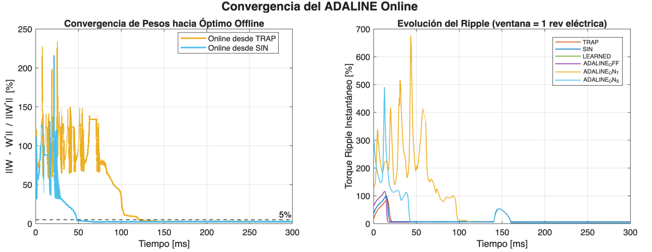
Figura 5.4: Convergencia del ADALINE en línea con observador. La señal de aprendizaje ruidosa vuelve el transitorio errático y más lento que en la figura 5.3: la inicialización senoidal cruza el 5 % hacia los 50 ms y la trapezoidal hacia los 120 ms. En régimen permanente ambas fluctúan por debajo del 5 % sin divergir.
