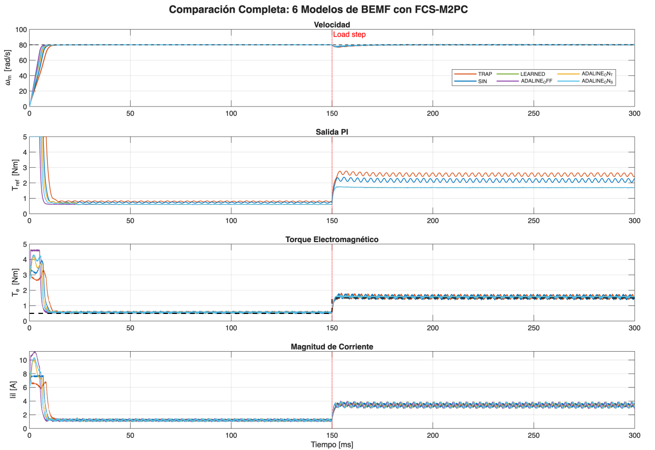
Figura 5.1: Corrida completa de los seis métodos con supervisión ideal: velocidad, salida del PI, par electromagnético y magnitud de corriente. El escalón de carga de 0,5 a 1,5 N·m entra en t = 150 ms. En las variables lentas los métodos son indistinguibles; las diferencias aparecen en la escala fina del par y de la salida del PI, donde TRAP y SIN oscilan visiblemente.
