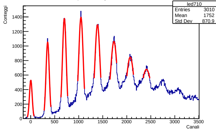
Spettro Digitaiser - 71.0V
