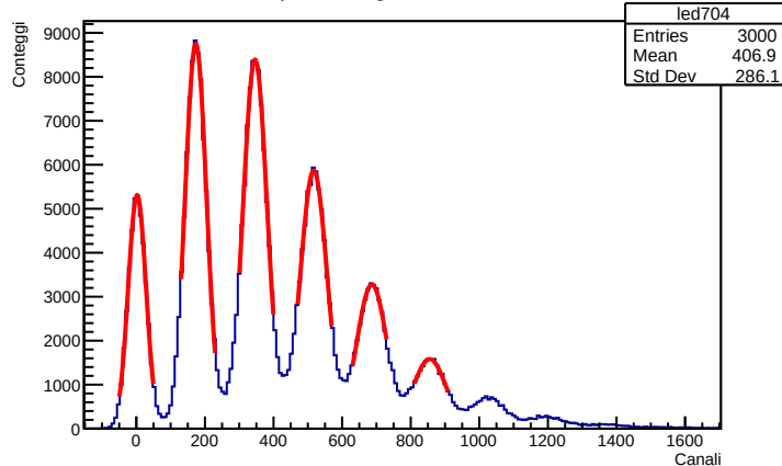
Spettro Digitaiser - 70.4V
