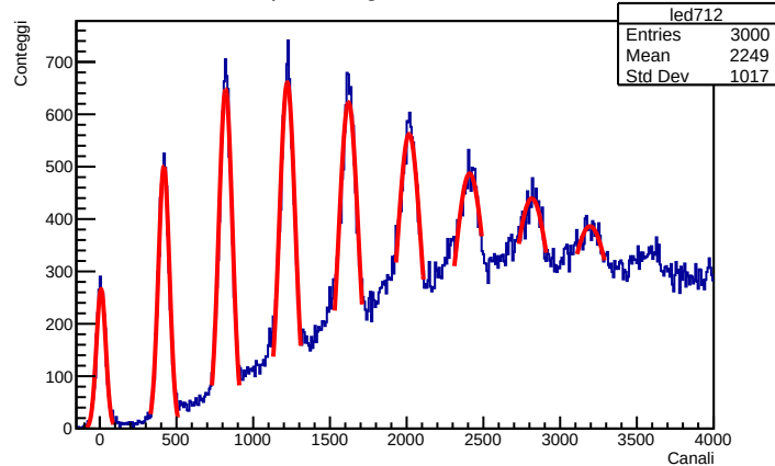
Spettro Digitaiser - 71.2V
