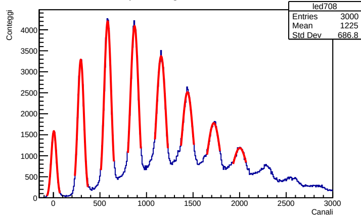
Spettro Digitaiser - 70.8V
