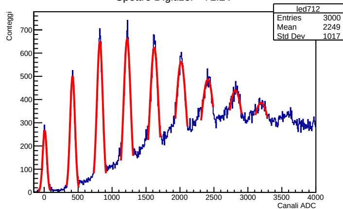
Spettro Digitizer - 71.2V
