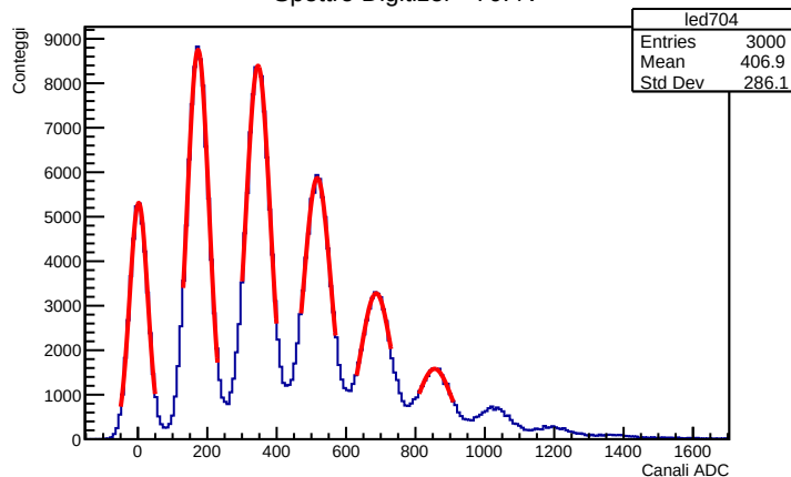
Spettro Digitizer - 70.4V
