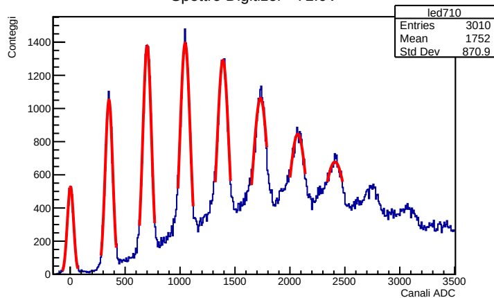
Spettro Digitizer - 71.0V
