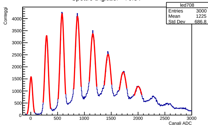
Spettro Digitizer - 70.8V
