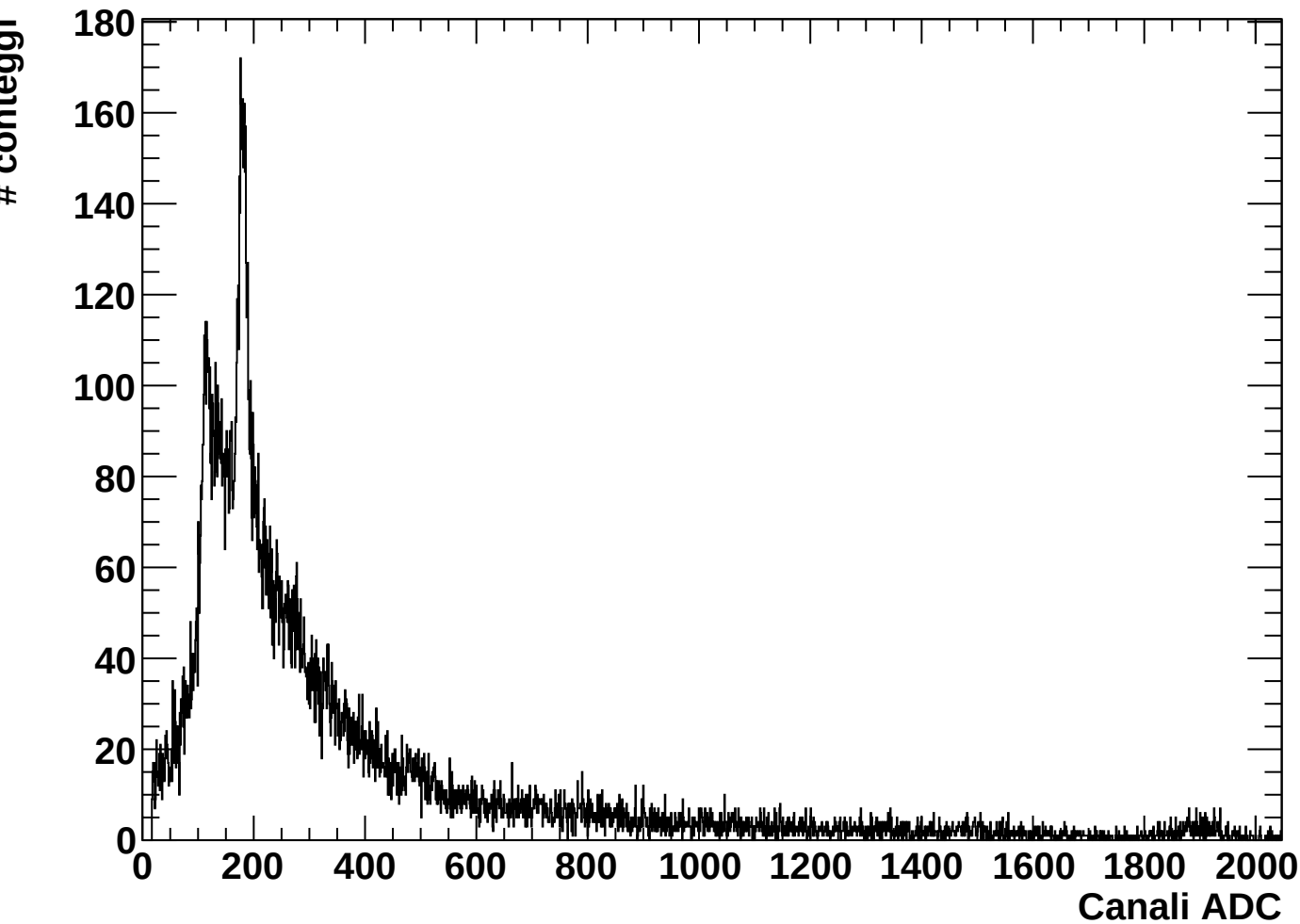
Spettro globale - Spettro_energia_ravvicinato_delay_ampl_0deg_Co57
