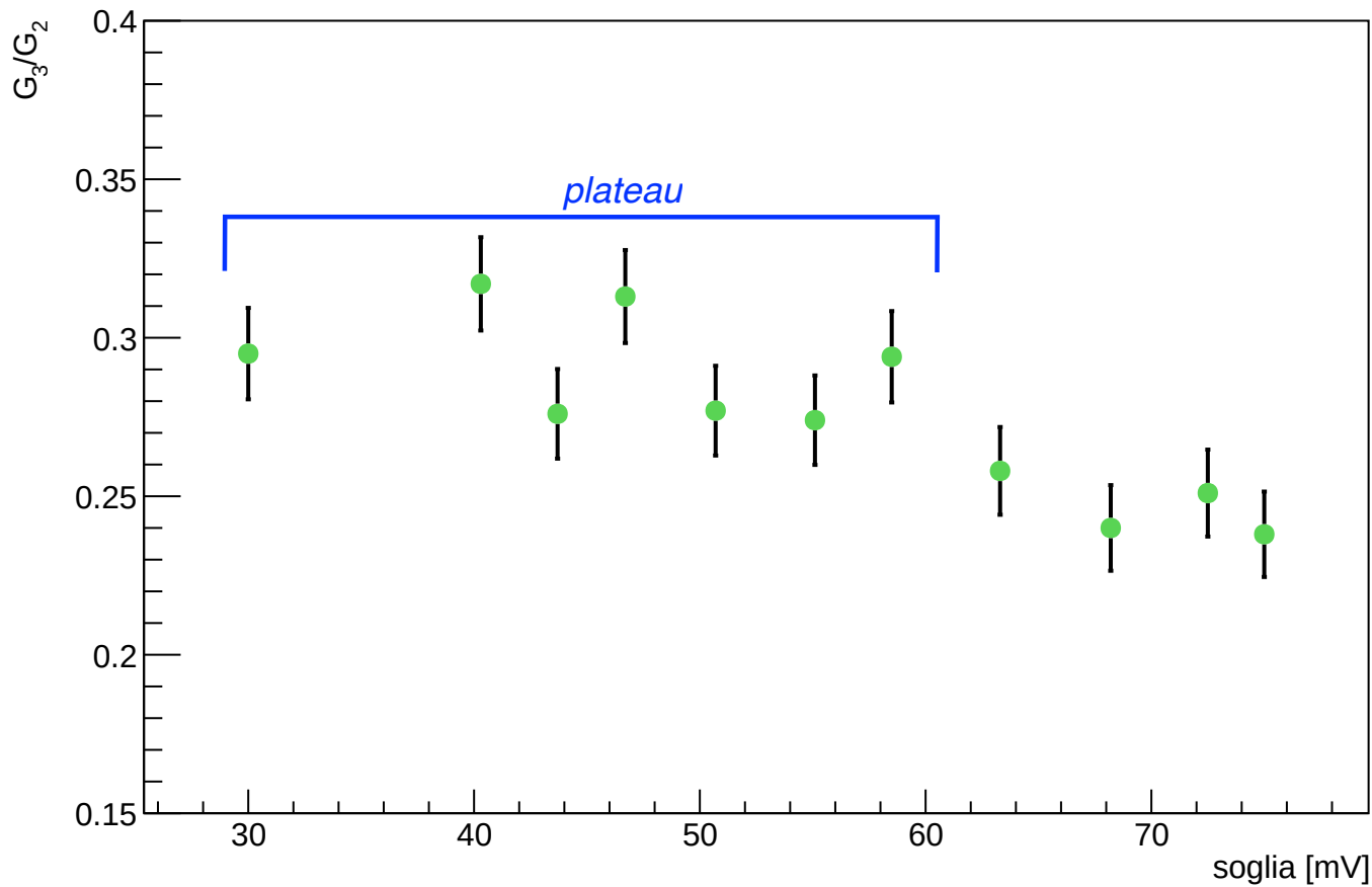
Frazione di eventi rivelati dallo scintillatore 8
