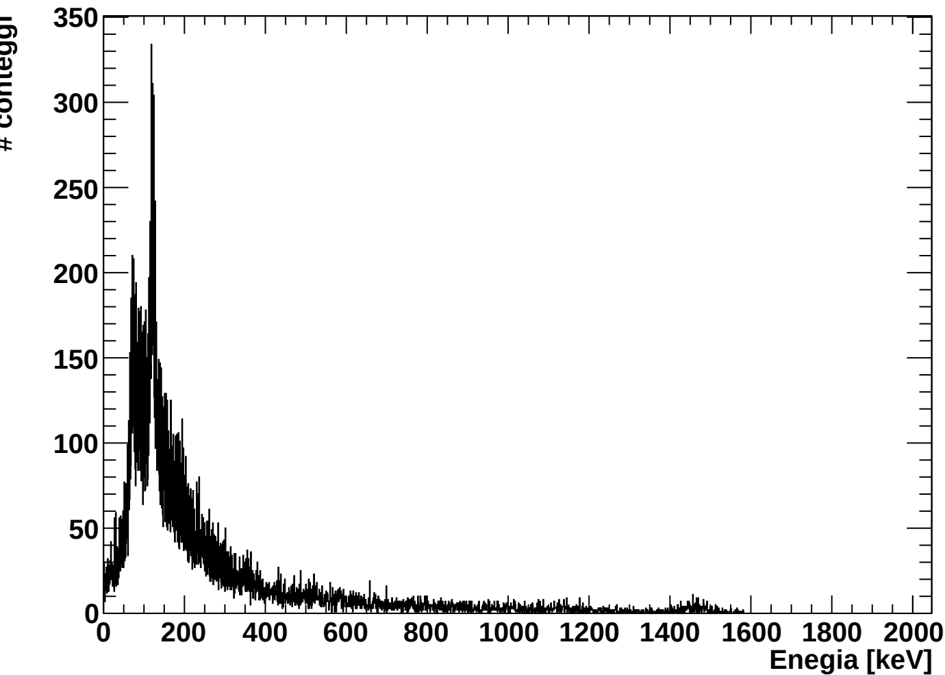
Spettro globale - Spettro_energia_ravvicinato_delay_ampl_0deg_Co57
