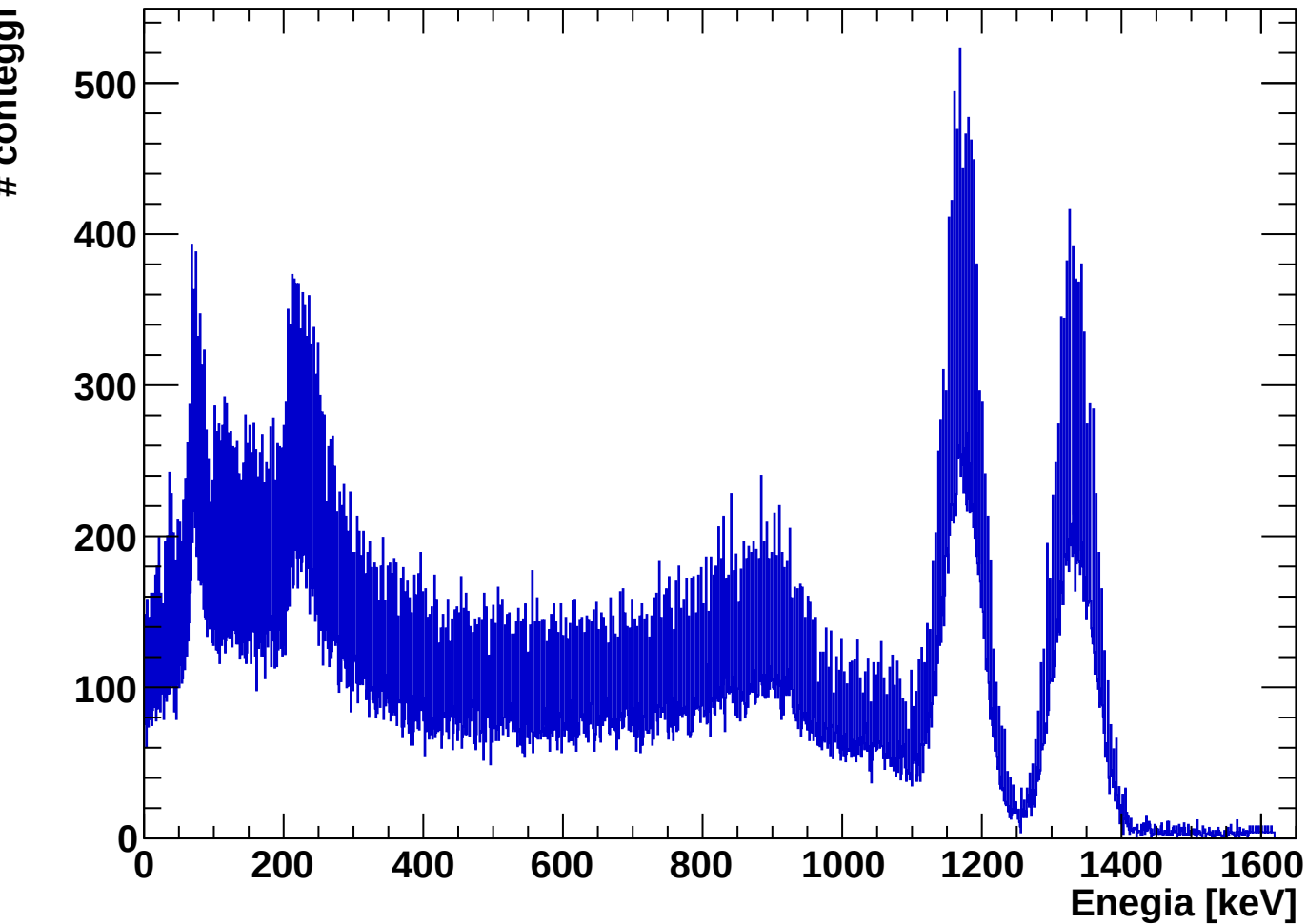
Spettro globale - Spettro_energia_ravvicinato_delay_ampl_0deg_Co60
