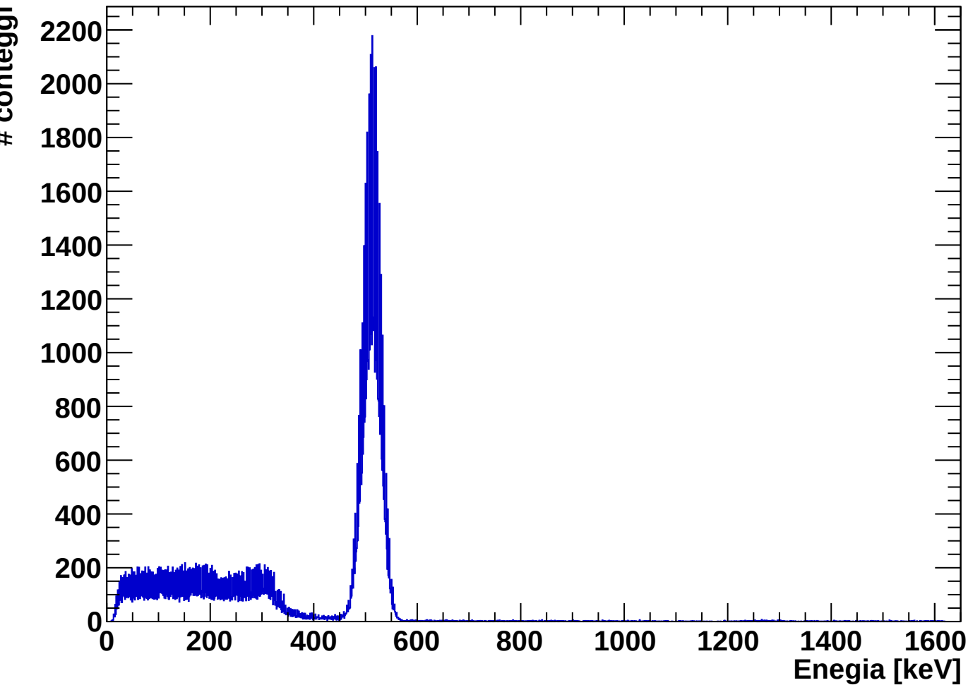
Spettro globale - Spettro_energia_trigger_mobile_0deg_Na
