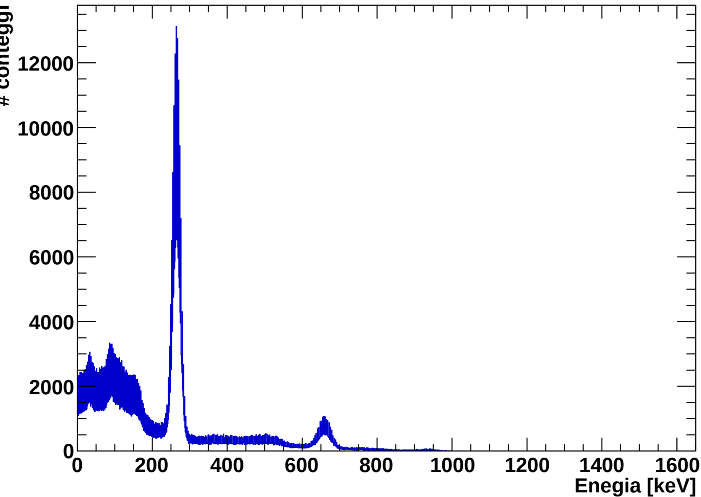
Spettro globale - Na_ravvicinatissimo_att20_withPb_piccosomma
