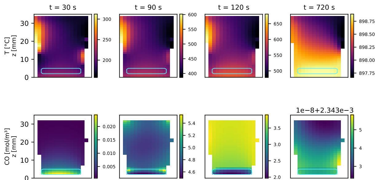
Figura 3: Corte vertical por el eje. Arriba la temperatura, abajo el CO; el contorno azul marca el lecho. Se ve la pastilla en el fondo y el frente térmico entrando por el cuerpo del crisol. A 720 s la escala de temperatura abarca poco más de un kelvin en todo el dominio.
