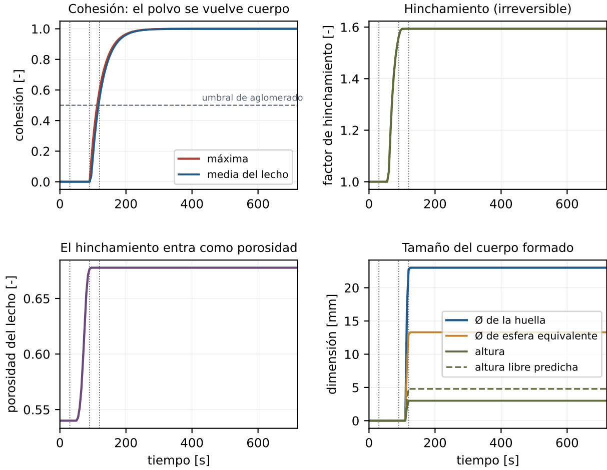
Figura 10: Formación del aglomerado. La cohesión cruza el umbral operativo hacia 115 s. El hinchamiento es irreversible: sube durante la etapa plástica y se queda.
