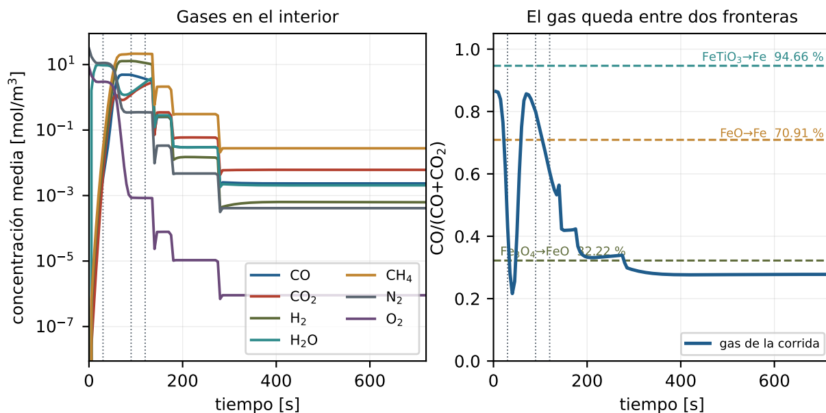
Figura 7: Izquierda: los gases del interior. Derecha: la razón \text{CO}/(\text{CO}+\text{CO}_2) frente a las tres fronteras. El gas se clava sobre la de la magnetita —no la cruza, se apoya en ella— y se queda muy lejos de la de la ilmenita. Ése es todo el argumento.
