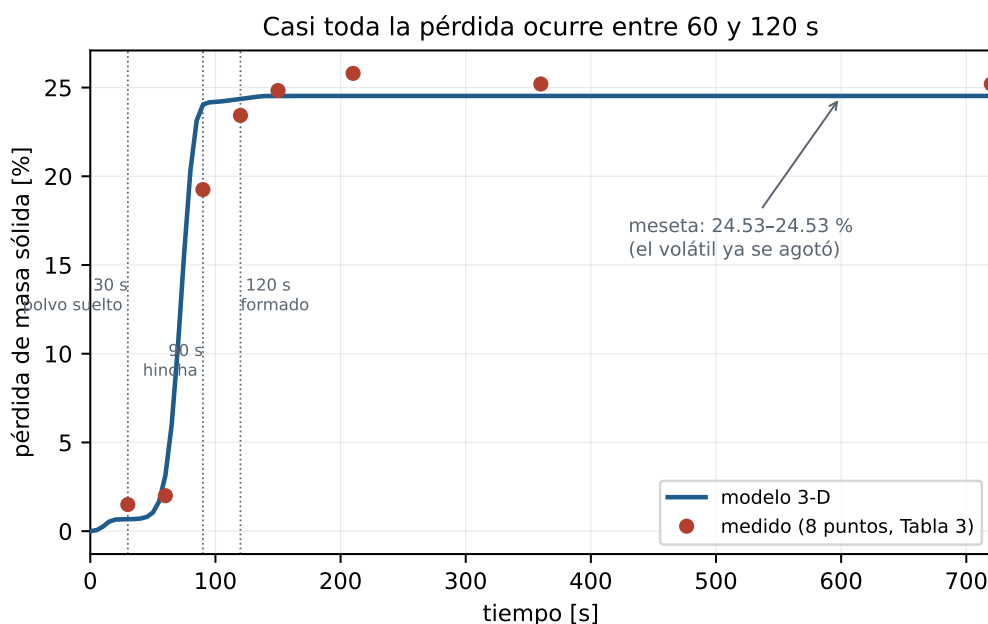
Figura 9: Pérdida de masa. La curva del modelo cae sobre los ocho puntos medidos sin haber sido ajustada a ellos.
