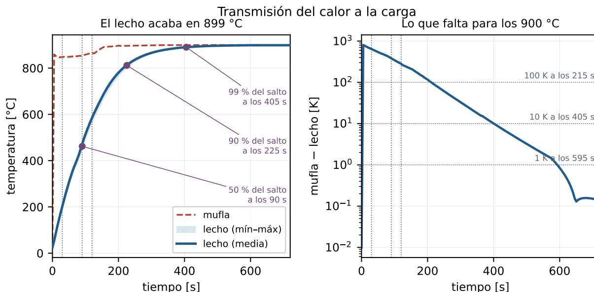
Figura 2: Transmisión del calor a la carga. A la izquierda, la temperatura media del lecho con su banda mínimo-máximo y los tres hitos del salto térmico. A la derecha, lo que le falta al lecho para alcanzar a la mufia, en escala logarítmica: si hubiese una sola constante de tiempo sería una recta, y no lo es, porque mientras dura la devolatilización el gas que sale se lleva calor y la pirólisis lo absorbe.
