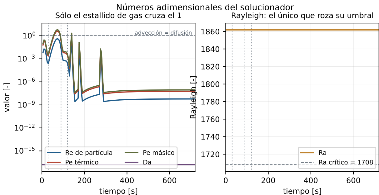
Figura 4: Evolución de los adimensionales. El pico hacia 75 s es la devolatilización: mientras el carbón suelta gas hay velocidad, y los Péclet suben más de cinco órdenes de magnitud y cruzan el 1. Fuera de esa ventana de unos treinta segundos vuelven a ser despreciables.
