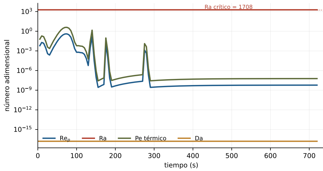
Figura 10: Números adimensionales calculados por el solucionador con las propiedades reales de cada celda. El colapso final de Re y Pe es el flujo apagándose cuando se agota el volátil: es un resultado, no un fallo. Da permanece en 10^{-17} : el transporte es órdenes de magnitud más rápido que la reacción.
