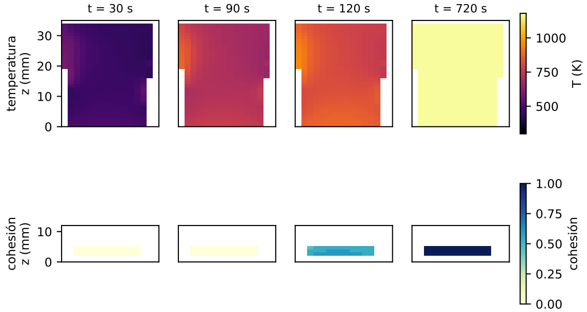
Figura 2: Cortes verticales por el eje del crisol. Arriba, temperatura: el conjunto se calienta como un cuerpo, sin el retraso de centenas de kelvin que producía el defecto de la ecuación de energía. Abajo, cohesión en el lecho.
