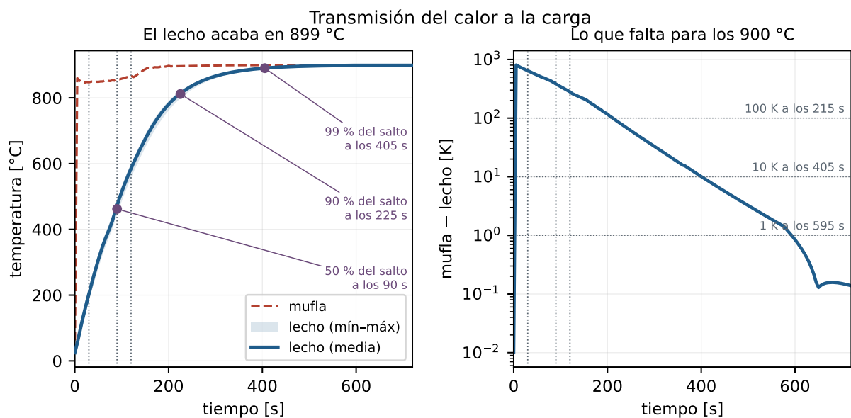
Figura 4: Transmisión del calor a la carga. A la izquierda, la temperatura media del lecho con su banda mínimo-máximo y los tres hitos del salto térmico. A la derecha, lo que le falta al lecho para alcanzar a la mufla, en escala logarítmica: si hubiese una sola constante de tiempo sería una recta, y no lo es, porque mientras dura la devolatilización el gas que sale se lleva calor y la pirólisis lo absorbe.
