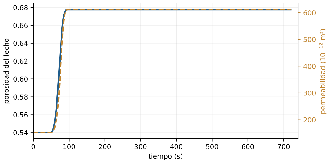
Figura 8: Porosidad del lecho y permeabilidad de Kozeny–Carman. Hasta esta revisión la porosidad estaba congelada en su valor inicial durante los 720 s, y con ella la permeabilidad, la conductividad efectiva y la tortuosidad de las difusividades.
