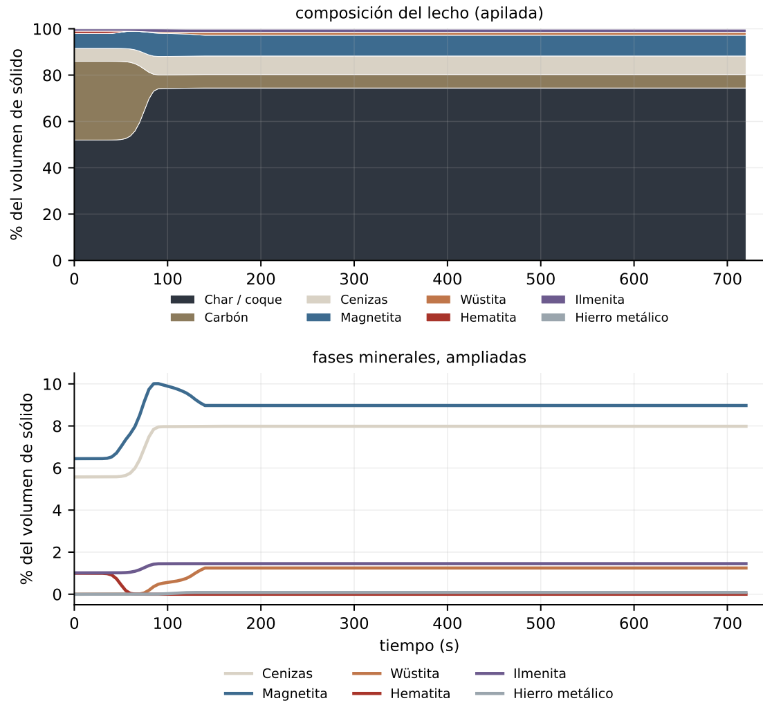
Figura 5: Composición del sólido del lecho en % de volumen. Arriba, apilada; abajo, las fases minerales ampliadas. Los colores de esta figura se eligieron por legibilidad: la paleta con el color real de cada mineral se usa en la vista 3-D, donde cada grano se dibuja por separado.
