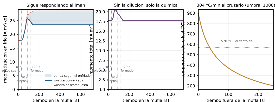
Figura 12: Izquierda: magnetización de saturación del lecho a temperatura ambiente, con la banda que abren los dos extremos del enfriado. Centro: el momento total, que no se entera de la dilución por pérdida de masa y sigue sólo a la química del hierro. Derecha: curva de enfriamiento del crisol al aire contra el eutectoide de la wüstita.
