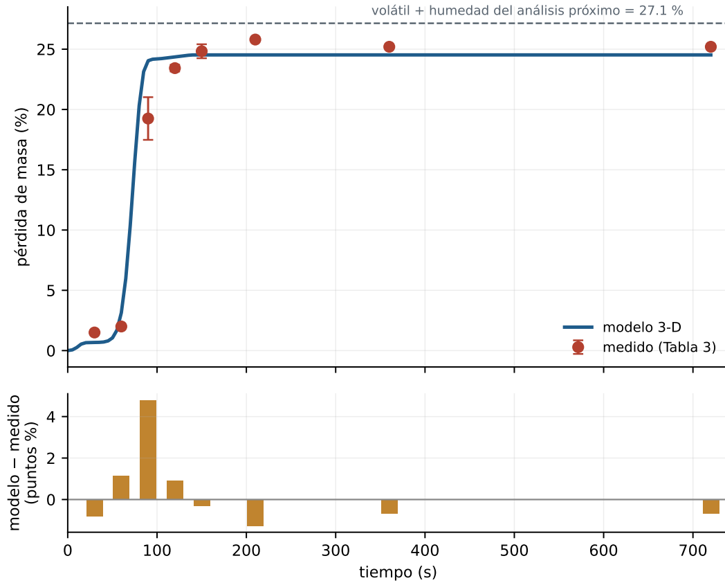
Figura 11: Pérdida de masa: modelo contra los ocho puntos medidos. Las barras son la desviación de las réplicas donde existen (los puntos de 30 y 60 s no la tienen). Abajo, el residuo punto a punto. La línea horizontal es el volátil más la humedad del análisis próximo: el máximo que el modelo puede perder por devolatilización.
