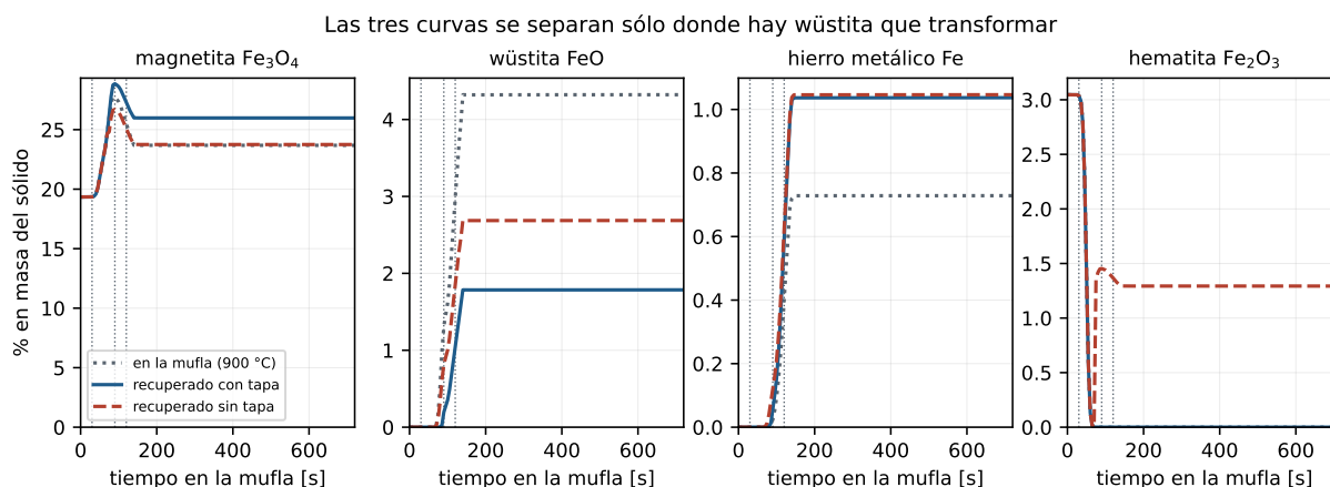
Figura 13: La misma fase en los tres estados en que puede encontrarse: dentro de la mufla, recuperada tras enfriar con la tapa puesta, y recuperada sin tapa. Las tres curvas nacen juntas y sólo se separan a partir de los 90 s, cuando aparece la primera wüstita: todo lo que distingue a las tres rutas —eutectoide, reoxidación por el gas encerrado, oxidación al aire— actúa sobre la wüstita o sobre lo que ella produce. Antes de que la haya, enfriar de una manera o de otra da exactamente el mismo sólido.
