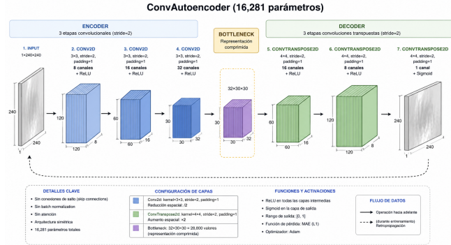
Figura 1: Arquitectura del autoencoder convolucional. El codificador reduce el corte cerebral con tres convoluciones de paso 2 hasta un cuello de botella de 30 \times 30 \times 32 ; el decodificador recupera la resolución original con convoluciones transpuestas. ReLU tras cada convolución, sigmoide a la salida.
