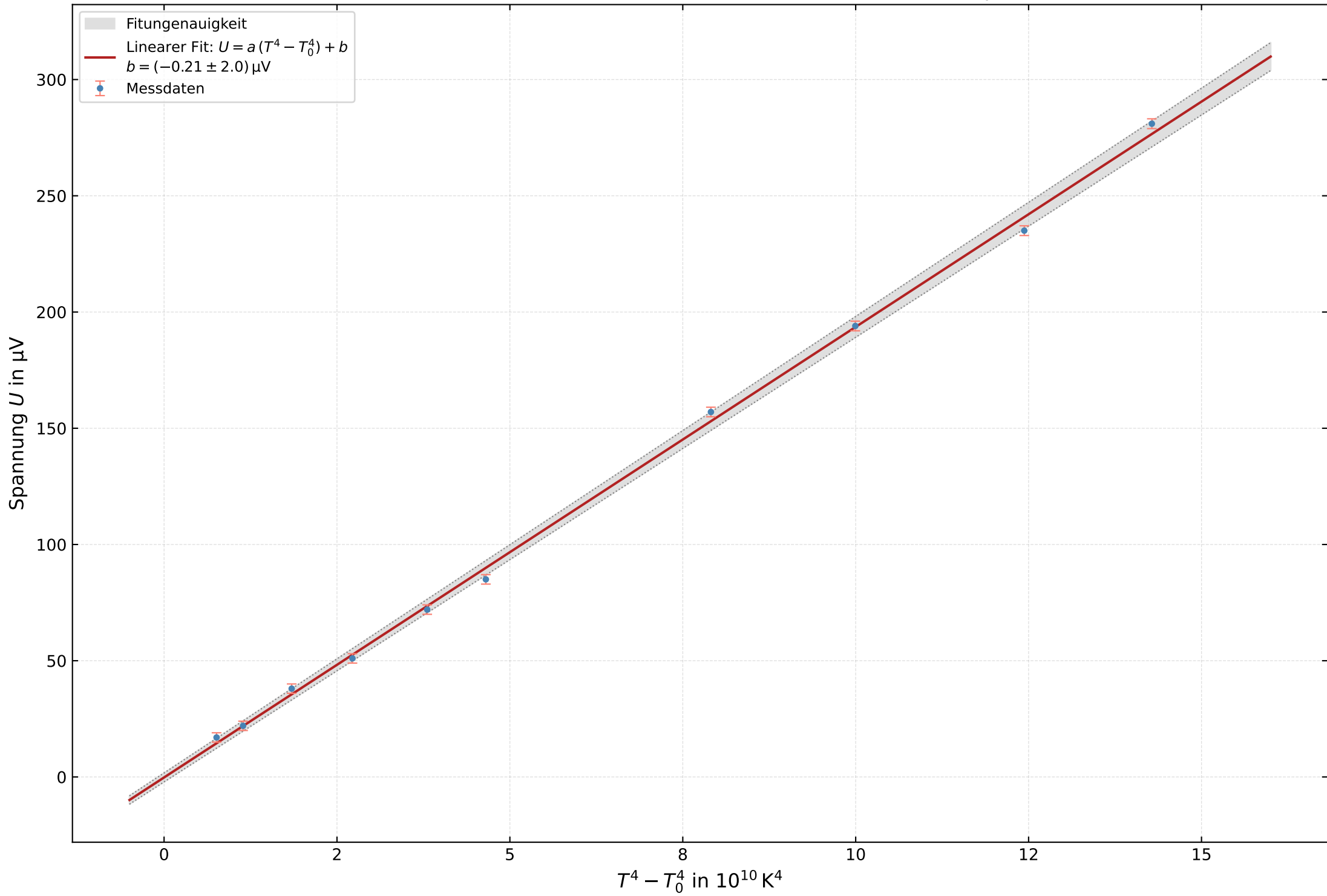
Spannung der Thermosäule in Abhängigkeit von T^4 - T_0^4
