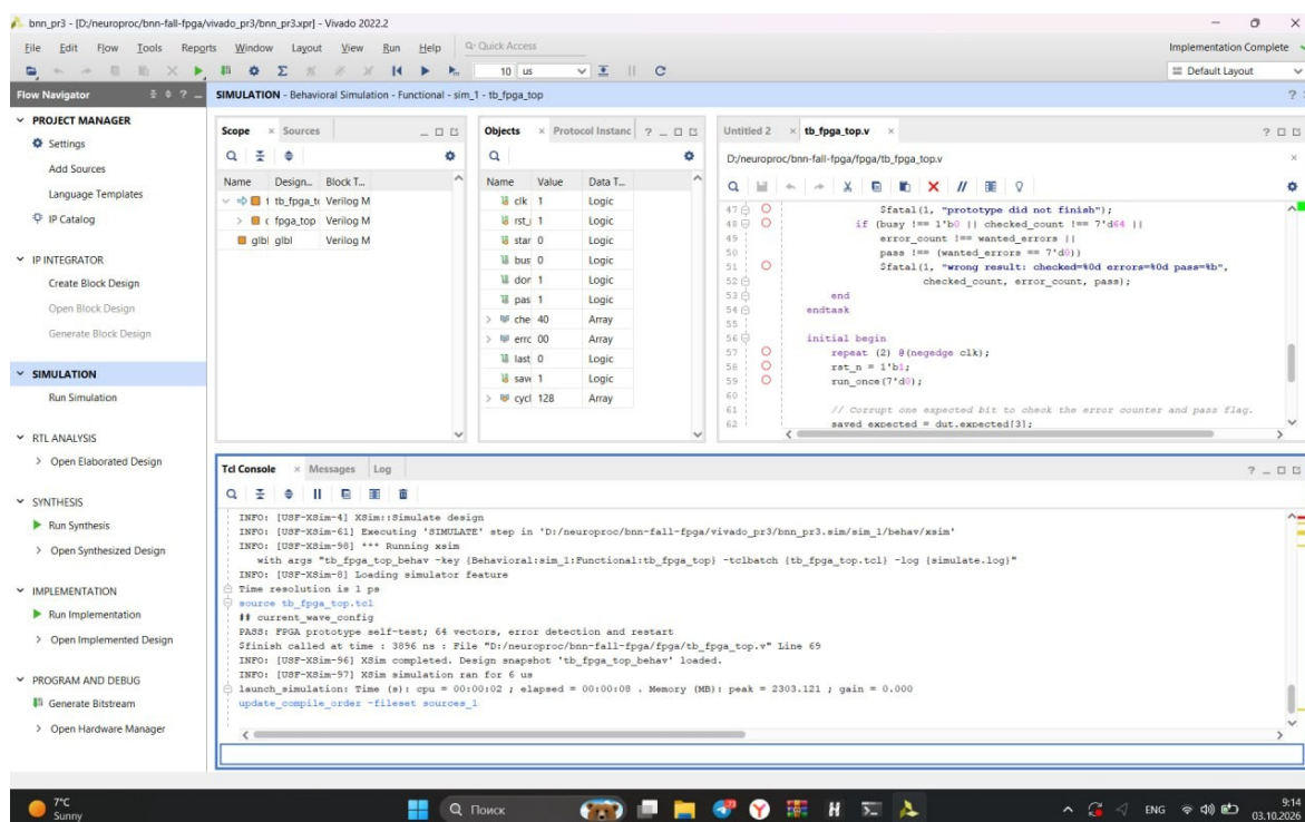
Рисунок 10.1 — Результат симуляции верхнего модуля в XSim
