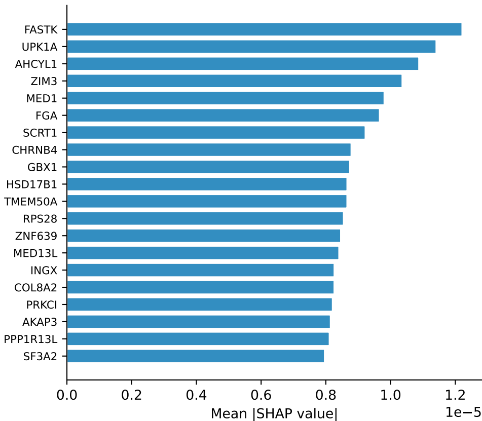
Top 20 geni per importanza media ProtoDANN — Test set (n = 23)
