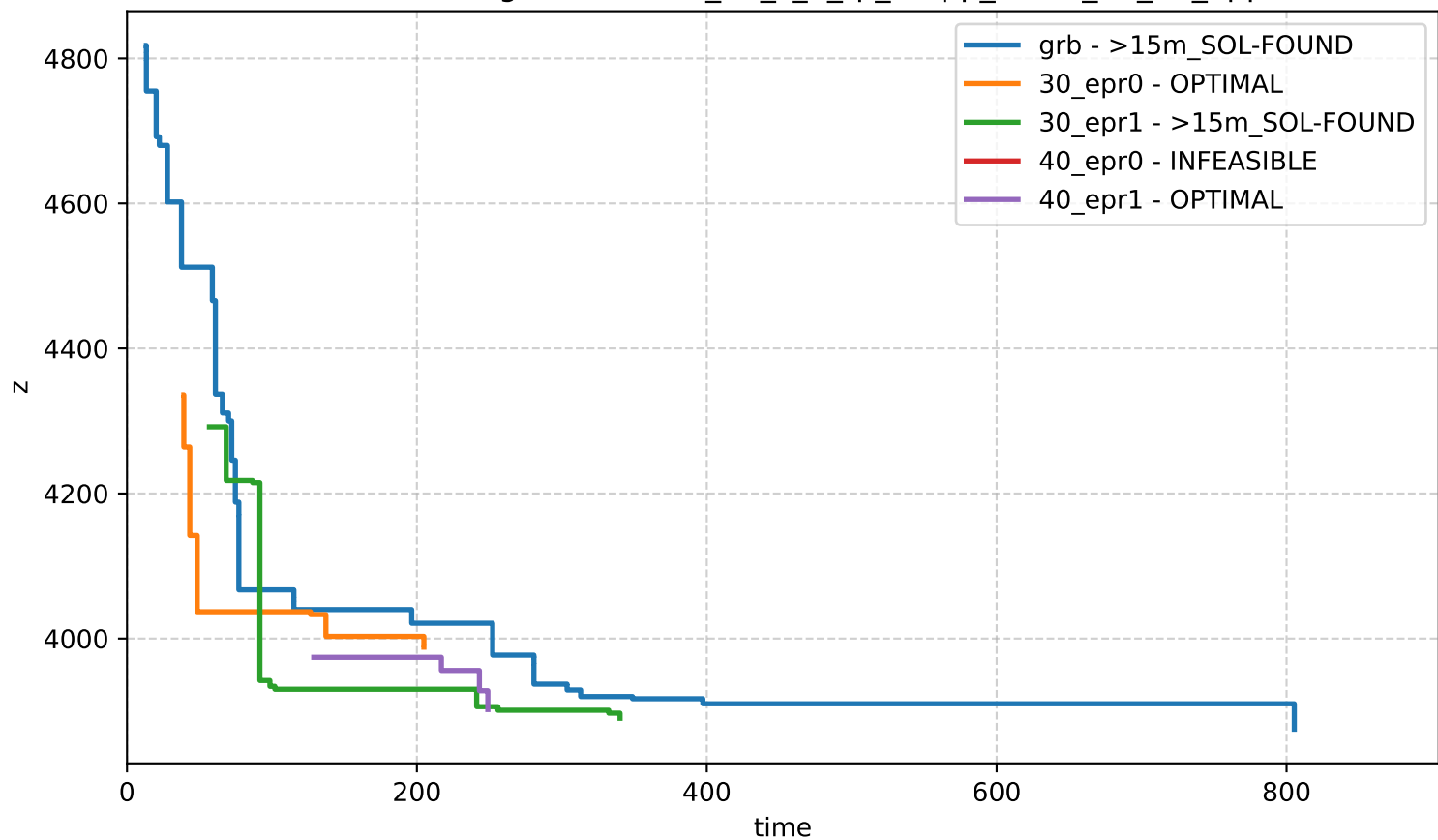
Bound Profiling - network-n_50_s_2_rp_0-app_set-id_37_17_apps
