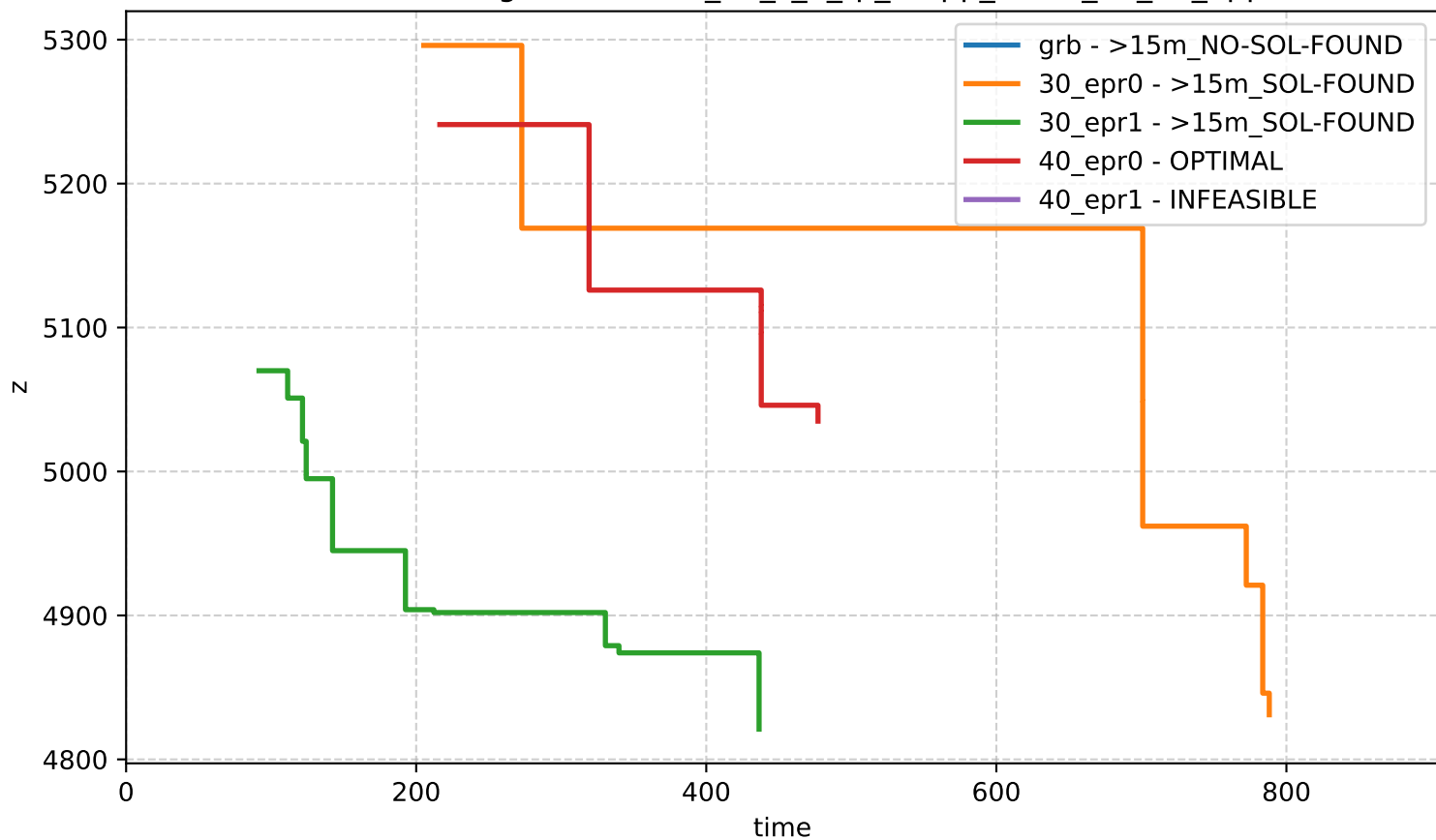
Bound Profiling - network-n_50_s_2_rp_0-app_set-id_36_17_apps
