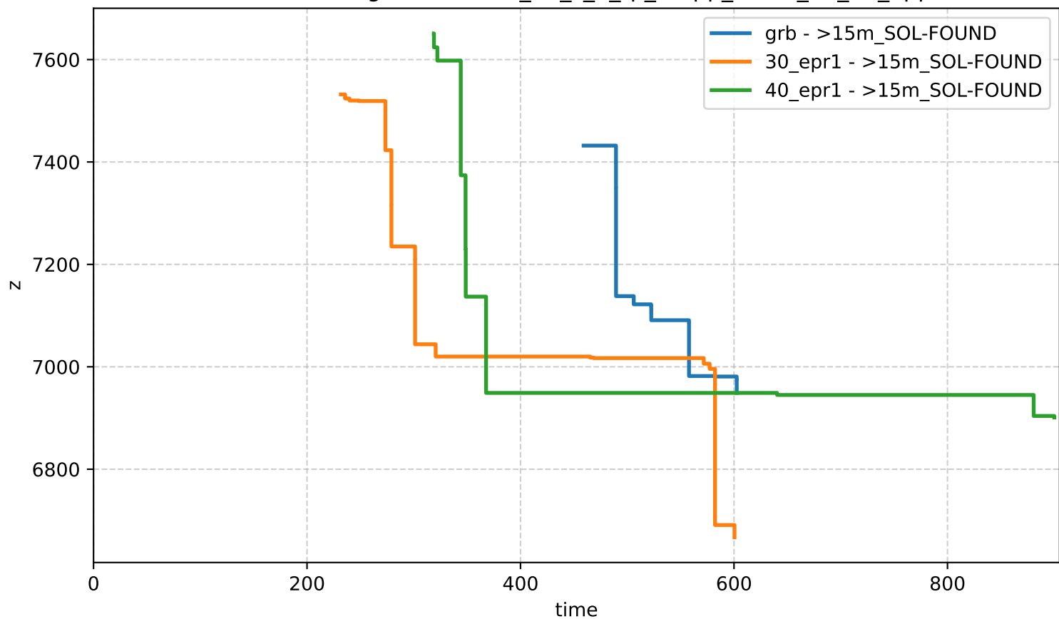
Bound Profiling - network-n_60_s_2_rp_0-app_set-id_67_27_apps
