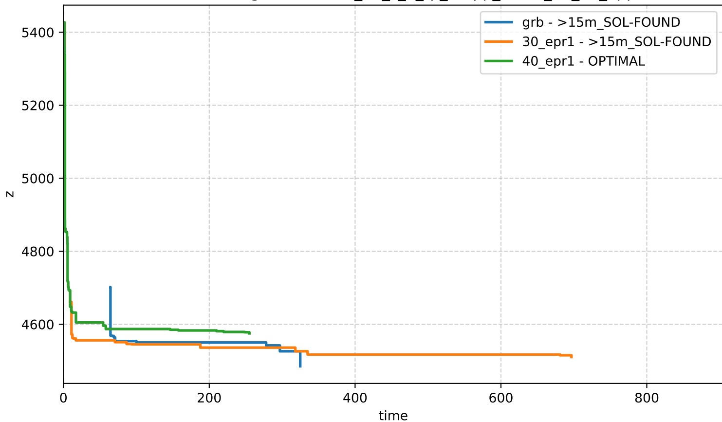
Bound Profiling - network-n_60_s_2_rp_0-app_set-id_40_18_apps
