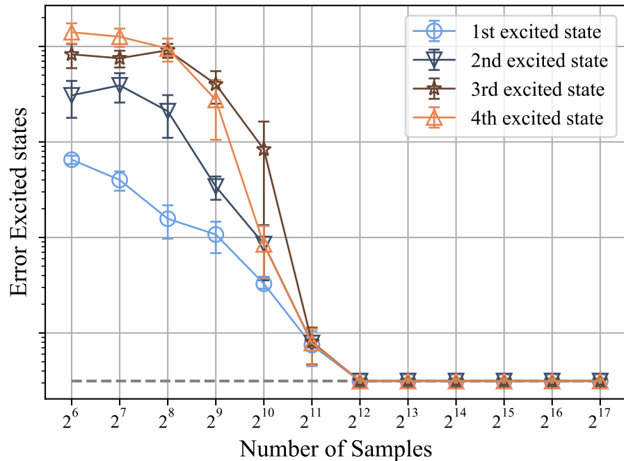
LiH (6-31G, R=1.5 \text{ \AA} , n_o = 10 , n_e = 4 )
