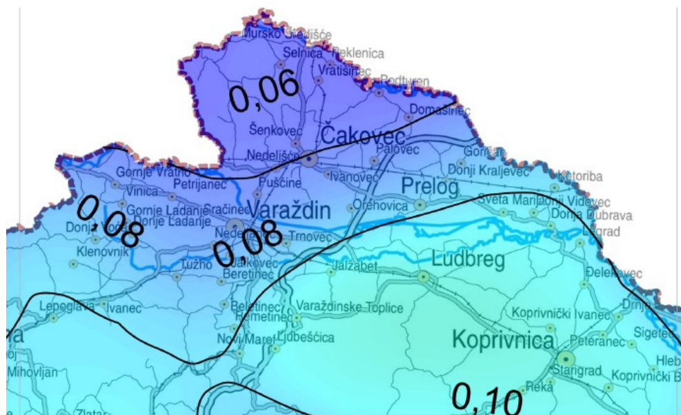
Slika 2: Karta potresnog područja s povratnim razdobljem od 95 godina za područje Županije
