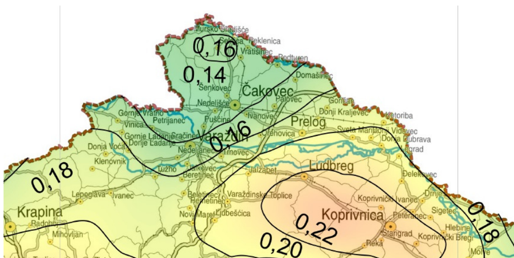
Slika 3: Karta potresnog područja s povratnim razdobljem za 475 godina za područje Županije
